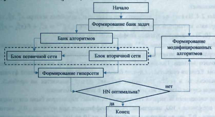
Рисунок 10 – Представление методов оптимизации в виде блок-схемы
