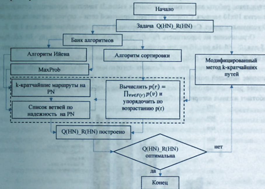
Рисунок 15 – Блок-схема модифицированного метода k-кратчайших путей
