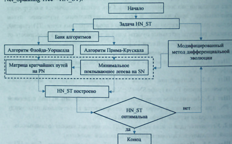
Рисунок 11 – Представление ММДЭ в виде блок-схемы
