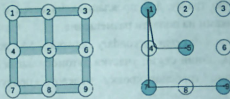
Рисунок 1 – Пример гиперсети
