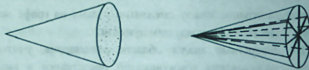
Рисунок 2 – Связность пар вершин в трехмерном пространстве а) Непрерывный случай б) Дискретный случай
