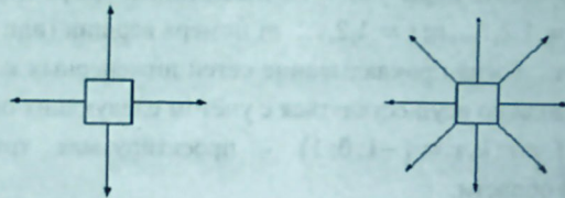
Рисунок 3 – Принципы связности точек в дискретном случае а) Четырехсвязность б) Восьмисвязность
