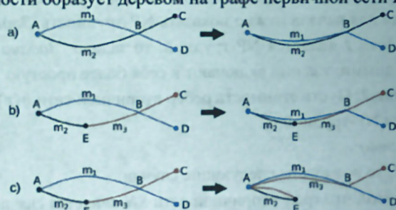
Рисунок 5 – Примеры маршрутов в графе первичной сети PN
