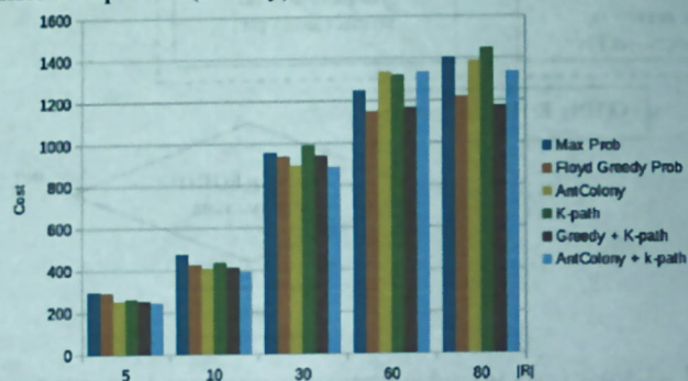
Рисунок 16 – Результаты работы алгоритмов для решетки 10 \times 10 , количество ребер вторичной сети от 5 до 80
