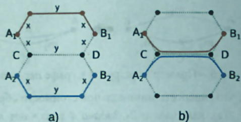
Рисунок 8 – Пример дерева Штейнера
