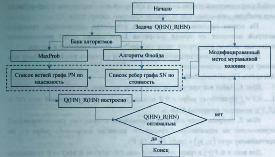
Рисунок 13 –Представление модифицированного AntColony в виде блок-схемы
