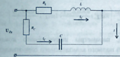
Рисунок 7 – Полная схема замещения индуктивного компонента
