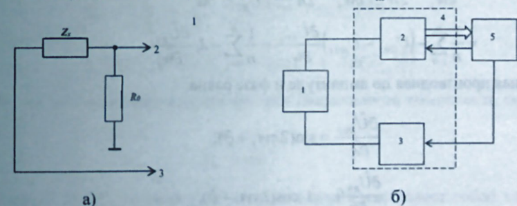
Рисунок 6 – Реализация измерителя параметров индукционных датчиков на базе устройства сбора данных Л Кард E502: а – принципиальная схема, б – структурная схема, 1-датчик, 2– АЦП, 3 – ЦАП, 4 – Л Кард E502, 5 – персональный компьютер.
