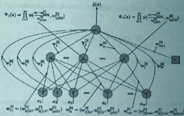
Рисунок 9 – Мультивейвлетная адаптивная сеть
