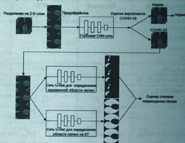
Рисунок 11 – Схема работы предлагаемой СИИ для диагностики COVID-19 по КТ-снимкам
