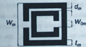
Рисунок 3 – Параметры CSRR ячейки-резонатора
