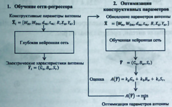
Рисунок 4 –Схема поиска оптимальной конструкции CSRR-ячеек микрополосковой антенны
