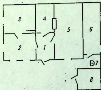
Рис. 4. План нового дома (1 — прихожая, 2—3 — спальни, 4 — летняя кухня, 5 — детская, 6 — зимняя кухня, 7 — навес, 8 — гараж)
