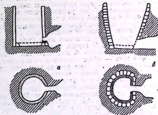
Рис. 1. Печи цилиндрической формы (а), печи в форме усеченного конуса с малым основанием внизу (б)
