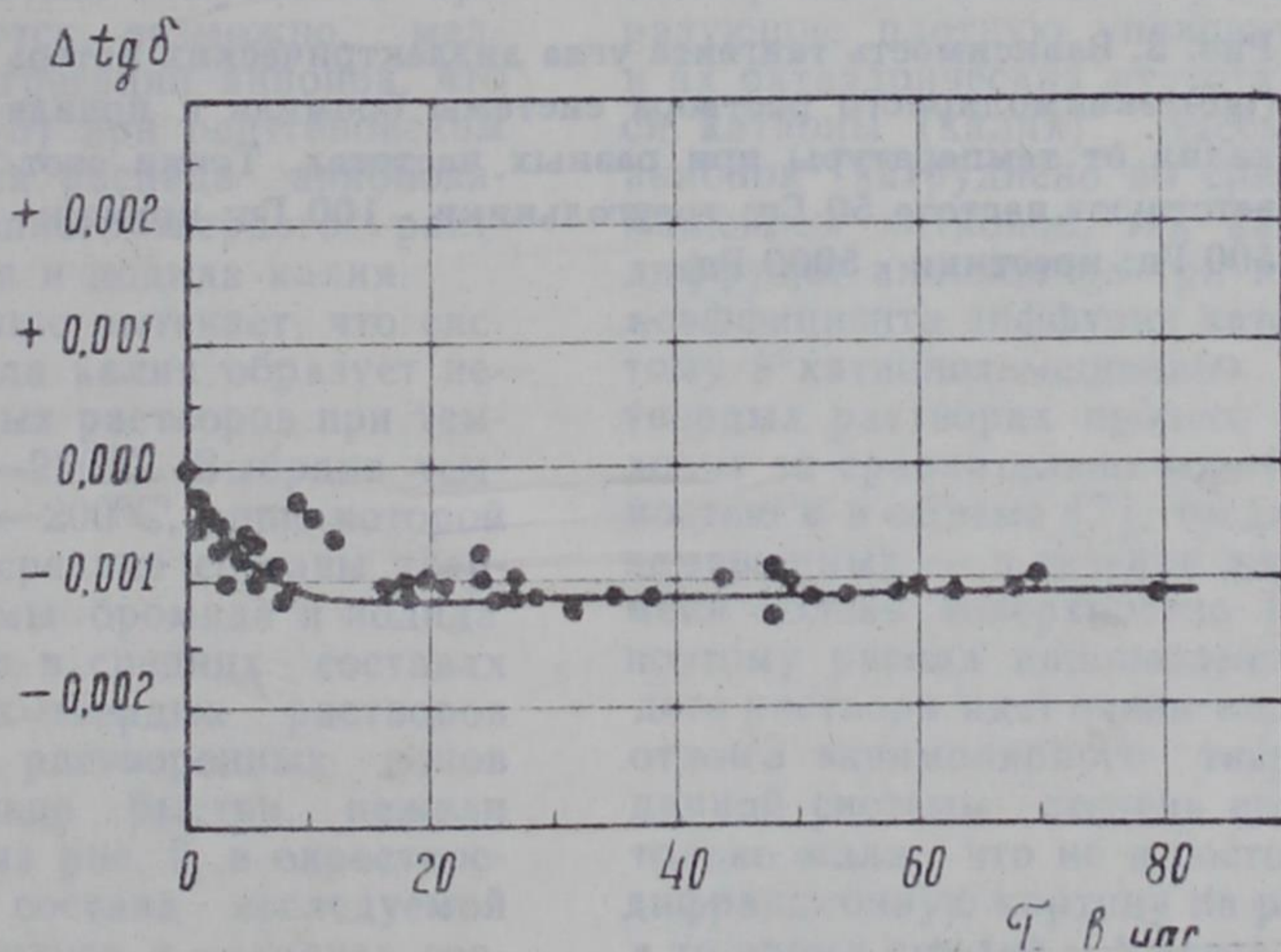
Рис. 2. Зависимость изменения тангенса угла диэлектрических потерь ( \Delta \text{tg} \delta ) эквимольного раствора системы бромида и иодида калия от времени изотермического отжига при 150°C. Частота измерения 100 Гц.
