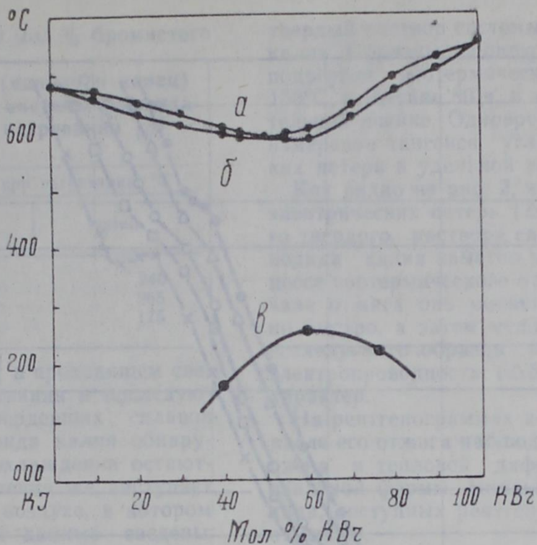
Рис. 1. Фазовые диаграммы бромида и иодида калия: а - кривая ликвидуса; б - кривая солидуса; в - кривая (сольвуса) растворимости компонент в твердом состоянии.
