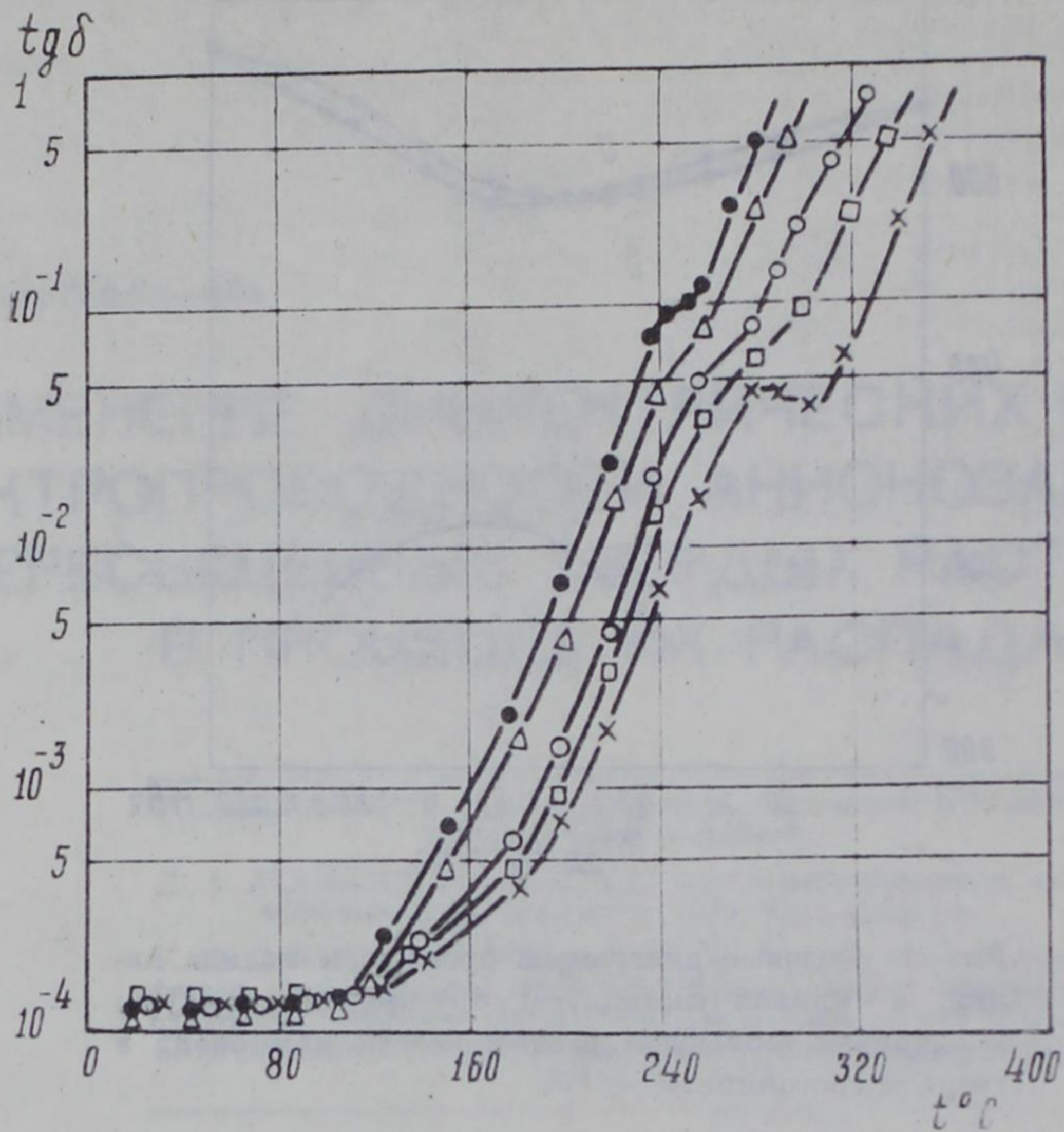
Рис. 3. Зависимость тангенса угла диэлектрических потерь ( \text{tg}\delta ) эквимольного раствора системы бромида и иодида калия от температуры при разных частотах. Точки соответствуют частоте 50 Гц; треугольники - 100 Гц; кружки - 500 Гц; крестики - 5000 Гц.
