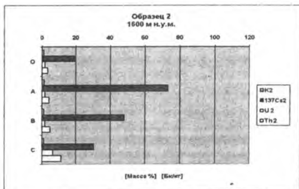
Рис. 3.8. Концентрация радиоактивных элементов в темно-каштановой почве.
