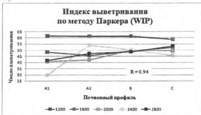
Рис. 3.3. Индекс выветривания по методу Паркера.
