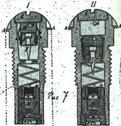
Рис. 7. Ударная трубка съ осядающимъ приспособленіемъ.
