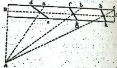
Фиг. 5. Определение места залегания фокуса по Маллету; de , fg , hk —направление трещин; A —фокус; Da , Db , Dc —длина распространения колебания.
