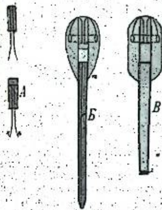
Рис. 10. Запалы Абеля пороховой (А) и гремучей (В).
