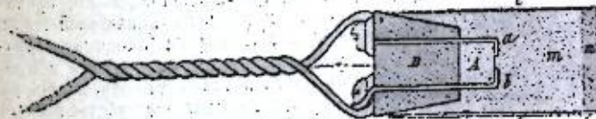
Рис. 13. Пробковый запал.
