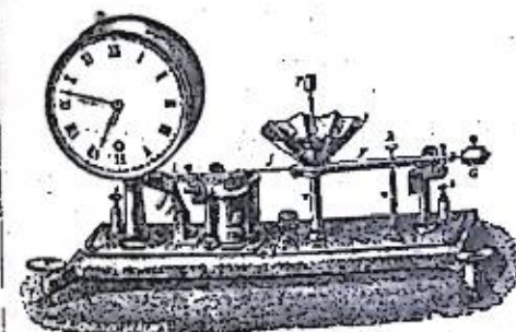
4. Указатель волнообразныхъ колебаній съ часами Брассера.
