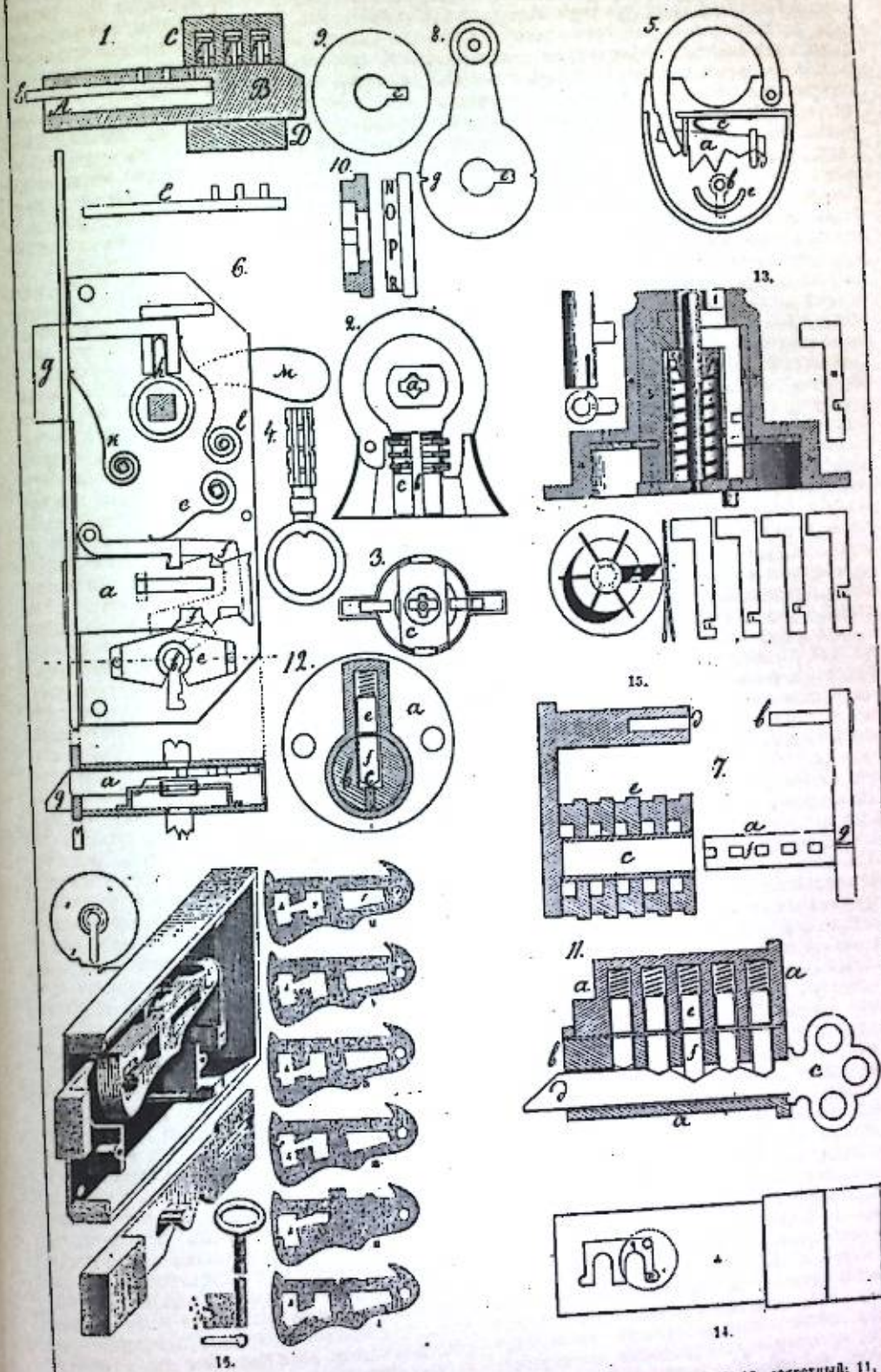
Замки: 1—древній египетскій; 2, 3, 4—шведскій; 5—французскій; 6—двойной; 7, 8, 9, 10—секретный; 11, 12—американскій; 13, 14, 15—Бранна; 16—Шубба.
