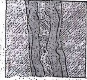
Рис. 5. Симметричное строение Ж. а — кварц, б — свинцовый блеск, в — известковый шпат, г — боковая порода.
