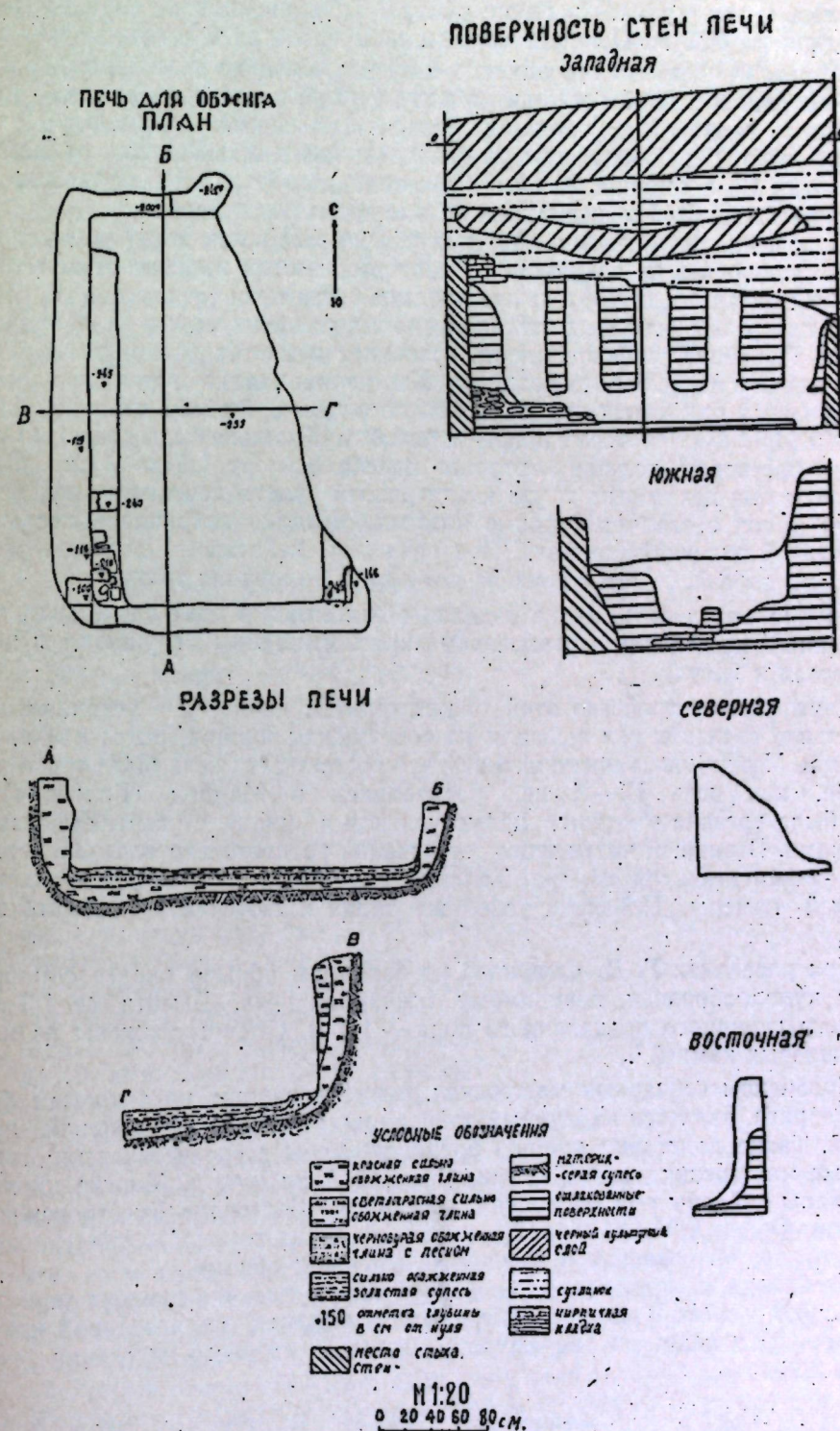
Рис. 5. Обжигательная печь (схема).
