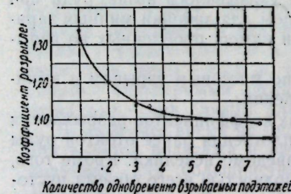
Рис. 1. Зависимость величины коэффициента разрыхления руды в блоке от количества одновременно взрываваемых подэтажей.
