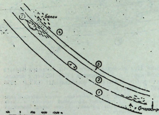
Рис. 2. Схема сопоставления разрезов роуксинского горизонта.
