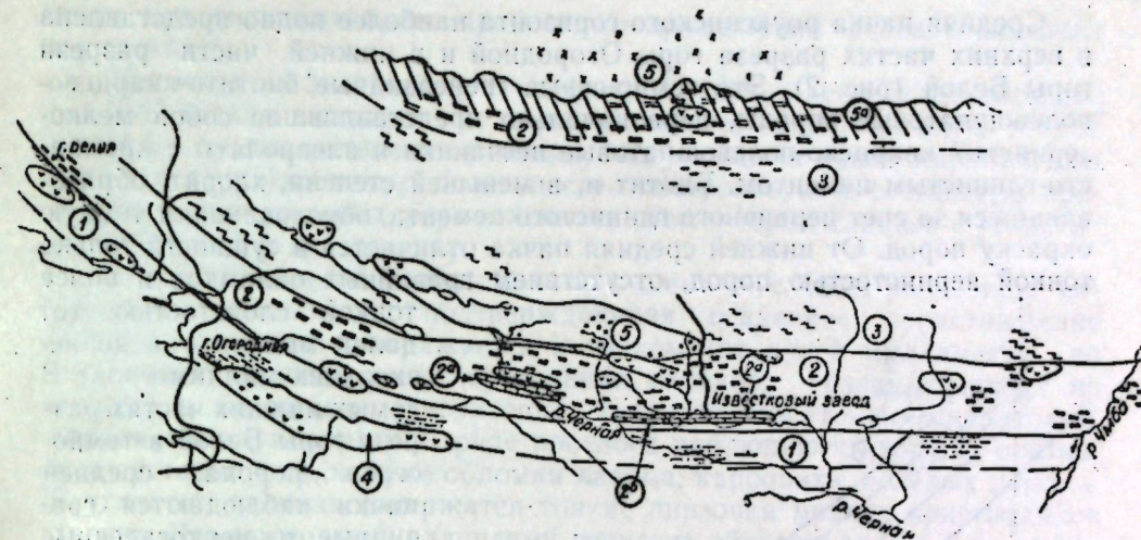
Рис. 1. Схема геологического строения Прихлебинской части свиты Имандра-Варзуга (составлена на основании геологической карты В. Е. Романова 1952—1953 гг. с использованием материалов геофизических работ Кольского филиала АН СССР 1956, 1935 и 1936 гг.).
