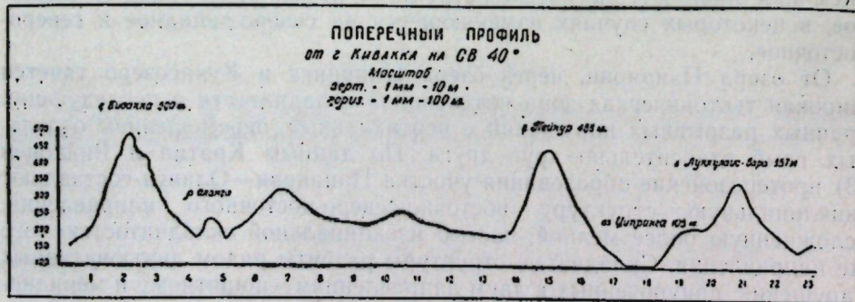
Рис. 1. Характер расчленения рельефа по линии г. Кивакка-Пяйнуур
