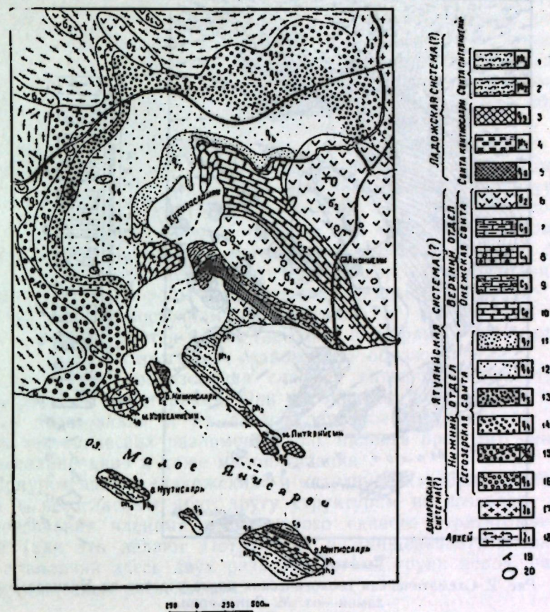
Рис. 1. Выкопировка из геологической карты района оз. М. Янисъярви, составленной Л. Н. Потрубович, О. Н. Анищенковой и др. в 1953—1956 гг.
