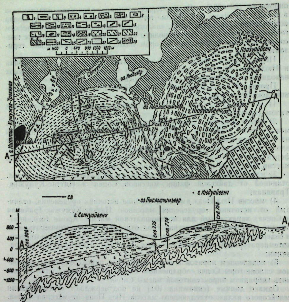
Рис. 1. Структурно-геологическая карта северо-восточной ветви Мончегорского плутона (по материалам Т. Н. Ивановой и Е. К. Козлова).
