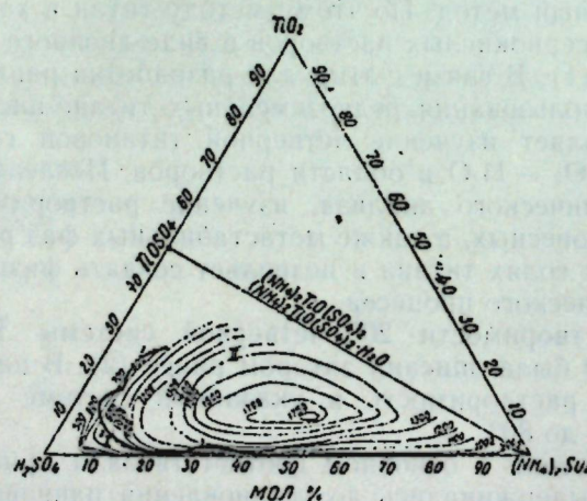
Рис. 1. Проекция изотермы растворимости системы \text{TiO}_2 - \text{H}_2\text{SO}_4 - (\text{NH}_4)_2\text{SO}_4 - \text{H}_2\text{O} при 0^\circ .
