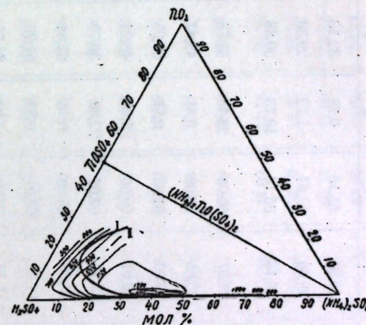
Рис. 4. Проекция изотермы растворимости системы \text{TiO}_2 - \text{H}_2\text{SO}_4 - (\text{NH}_4)_2\text{SO}_4 - \text{H}_2\text{O} при 80^\circ .
