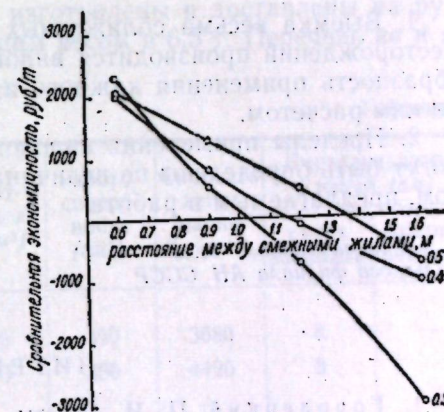
Рис. 2. Сравнительная экономичность валовой выемки сближенных жил по отношению к раздельной.
