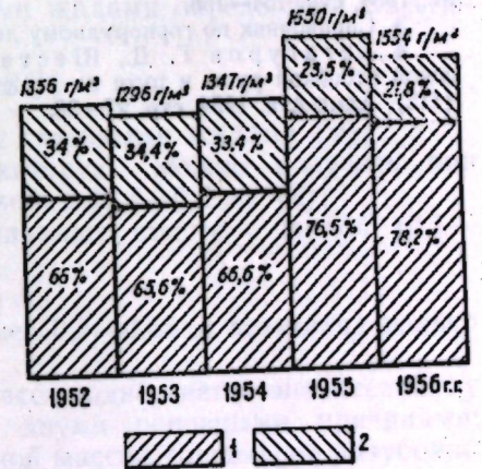
Рис. 4. Диаграмма соотношения удельных расходов вв на отбойку и вторичное дробление и выпуск руды на апатитовом руднике им. С. М. Кирова. 1—удельный расход вв на отбойку; 2—удельный расход вв на вторичное дробление и выпуск руды.
