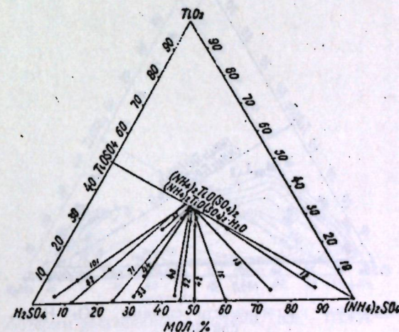
Рис. 2. Определение солевого состава двойных солей методом остатка при 0^\circ .
