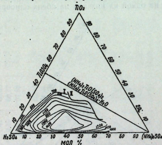
Рис. 3. Проекция изотермы растворимости системы \text{TiO}_2 - \text{H}_2\text{SO}_4 - (\text{NH}_4)_2\text{SO}_4 - \text{H}_2\text{O} при 40^\circ .
