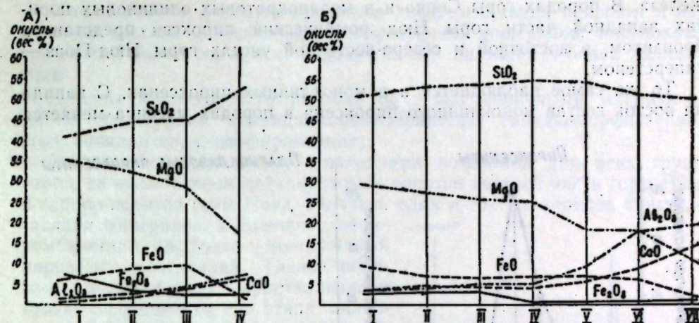
Рис. 2. Вариационные диаграммы. Римскими цифрами на диаграммах обозначены средние содержания окислов в различных группах пород.
