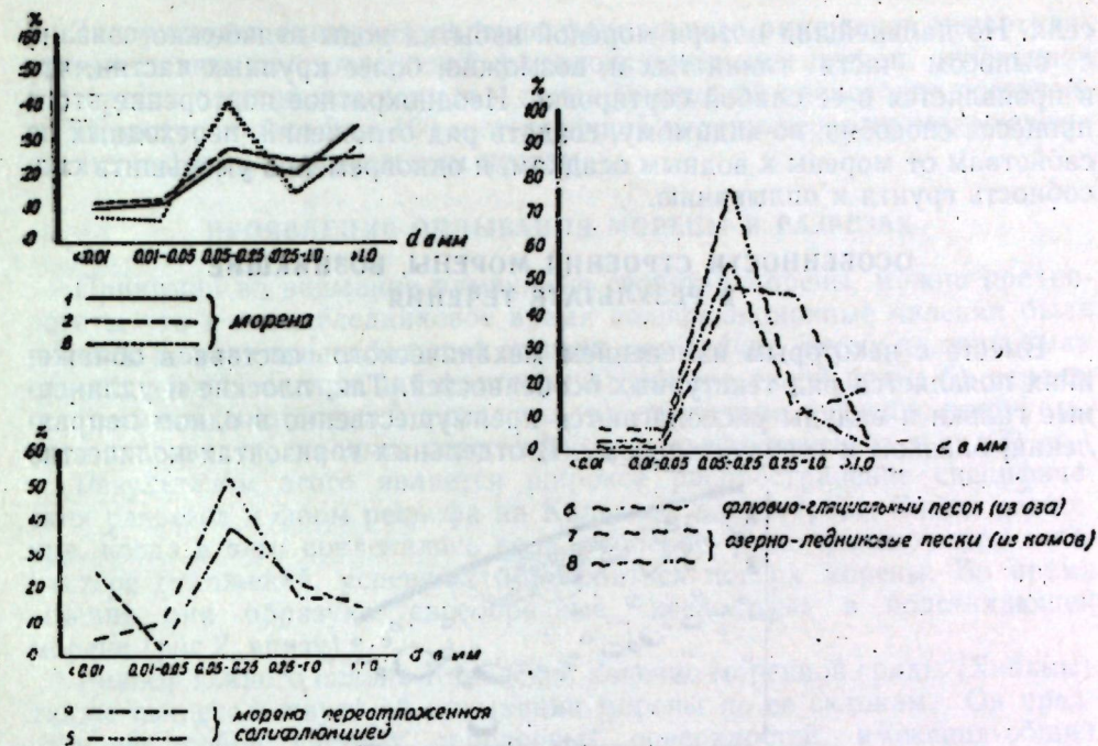
Рис. 1. Суммарные кривые различных типов ледниковых отложений.
