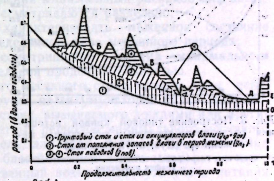
Рис. 2. Схематический гидрограф межени и его составляющие.
