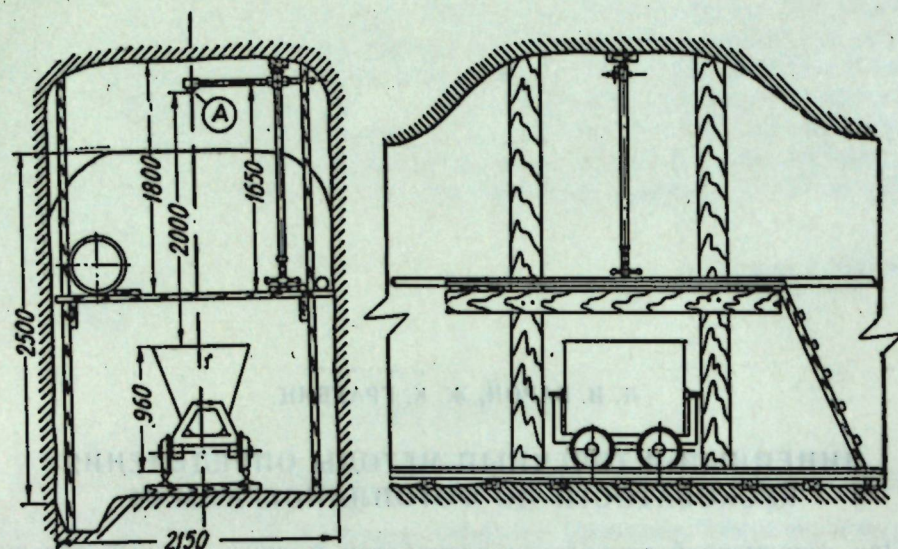
Рис. 1. Установка для фотографирования породы в вагонетках.
