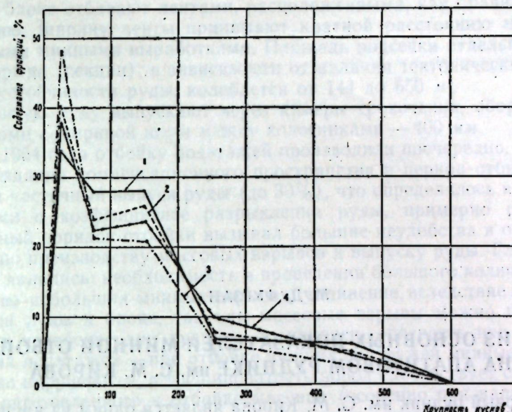
Рис. 2. Кривые гранулометрического состава отбитой породы при опытах на руднике «Ниттис-Кумужье».
