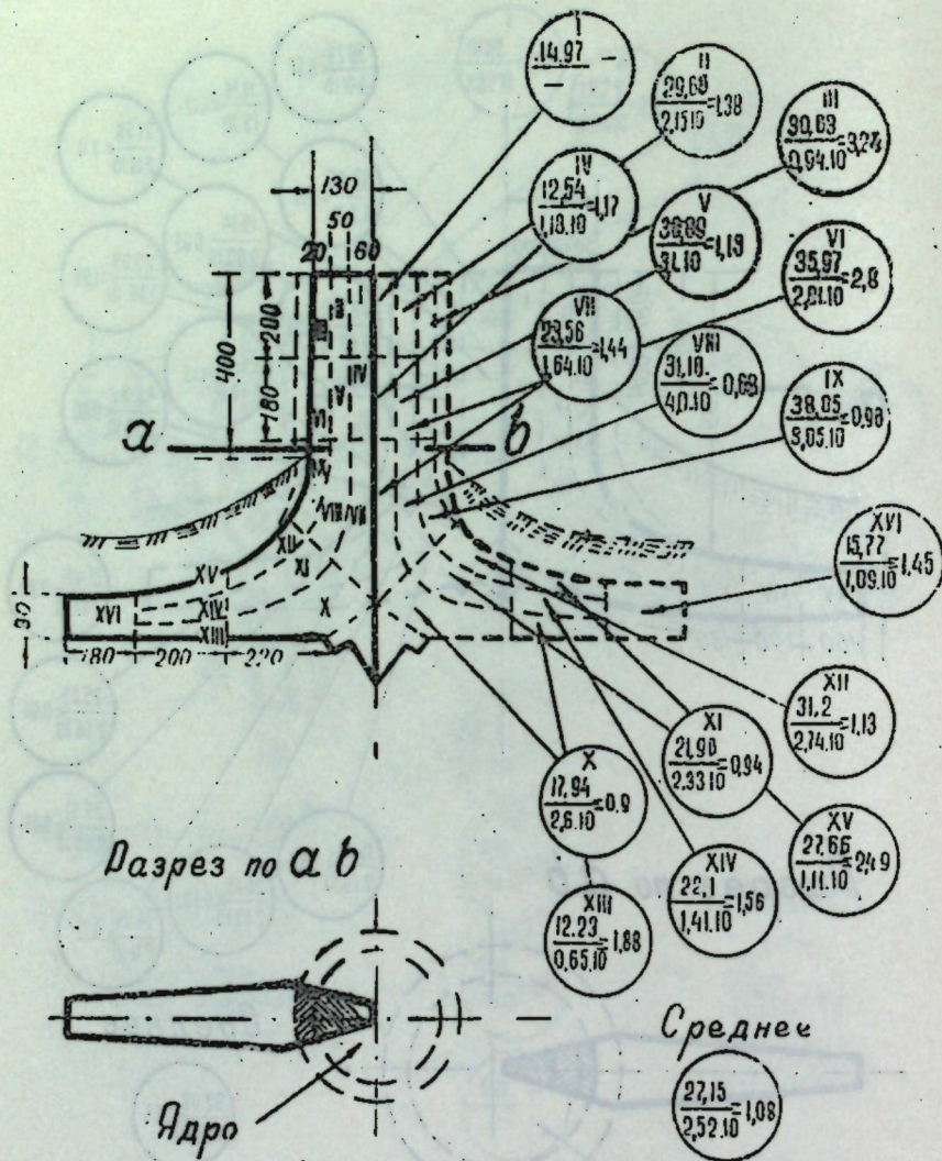
Схема распределения смолы и скипидара в сосновом пне. Образец № 5, взятый в Пряжнинском р-не, пос. Матросы. Год рубки 1920. Год корчевки 1919.
