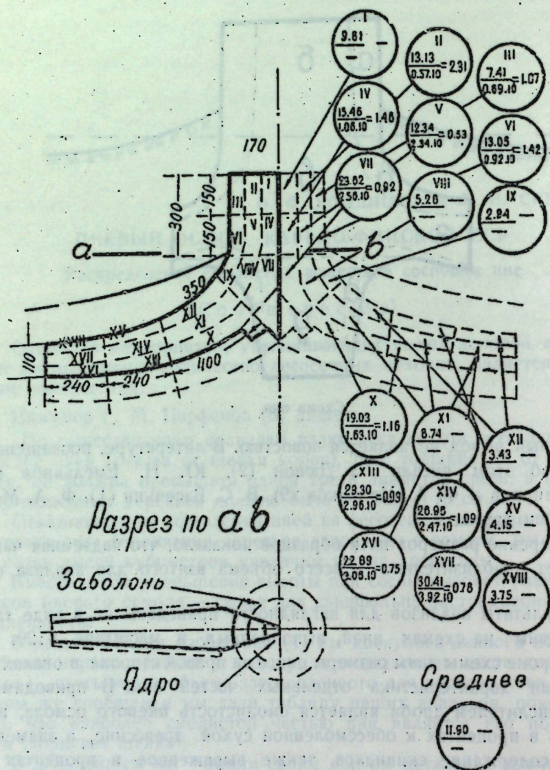
Схема распределения смолы и скипидара в сосновом пне. Образец № 1, взятый в Пляжинском р-не, пос. Матросы. Год рубки 1949. Год корчевки 1949.
