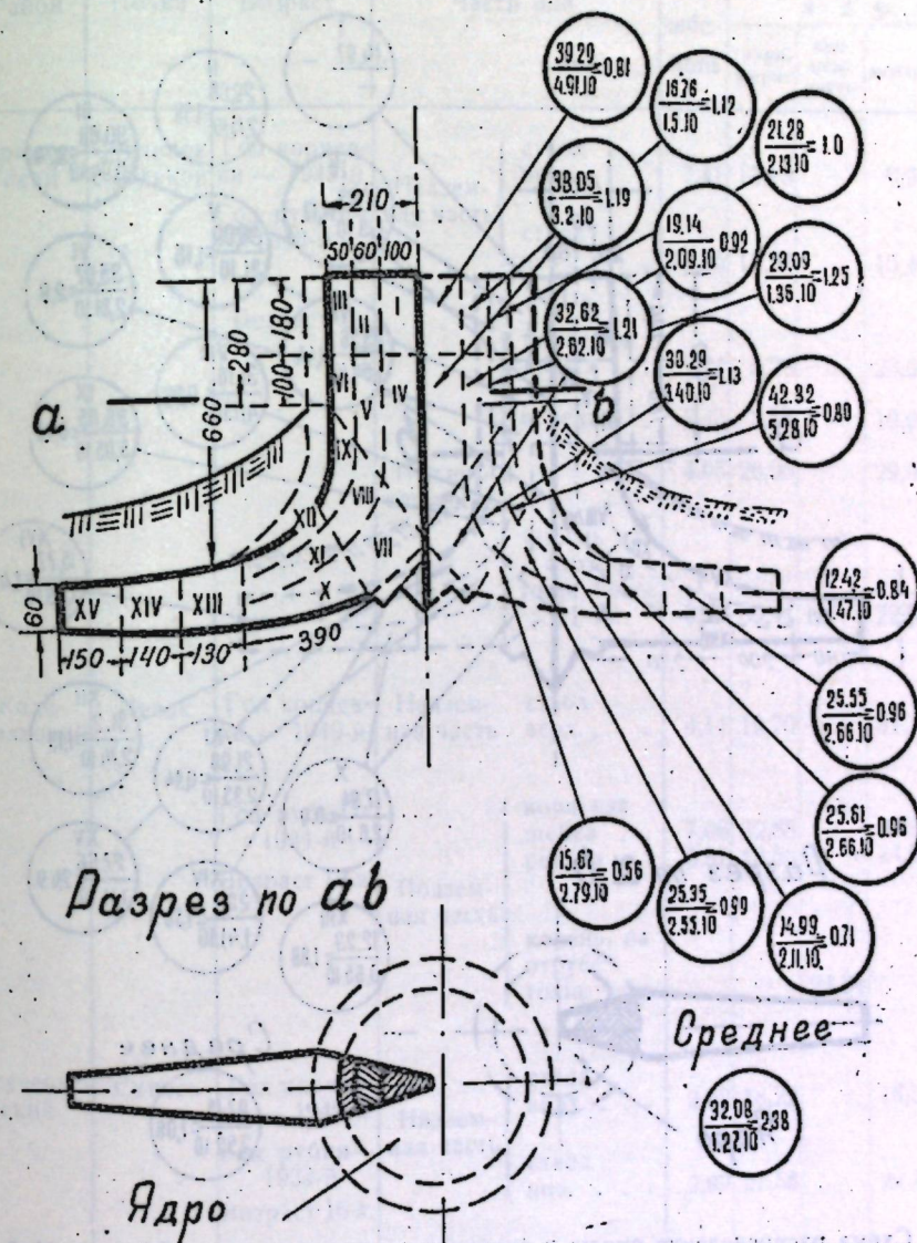
Схема распределения смолы и скипидара в сосновом пне. Образец № 4, взятый в Пряжинском р-не, пос. Матросы. Год рубки 1920. Год корчевки 1949.
