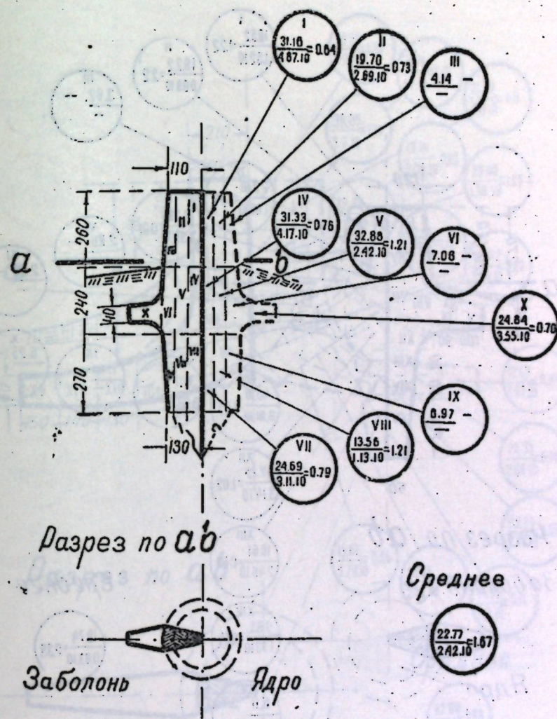
Схема распределения смолы и скипидара в сосновом пне. Образец № 2, взятый в Калевальском р-не, село Ухта. Год рубки 1934. Год корчевки 1949.
