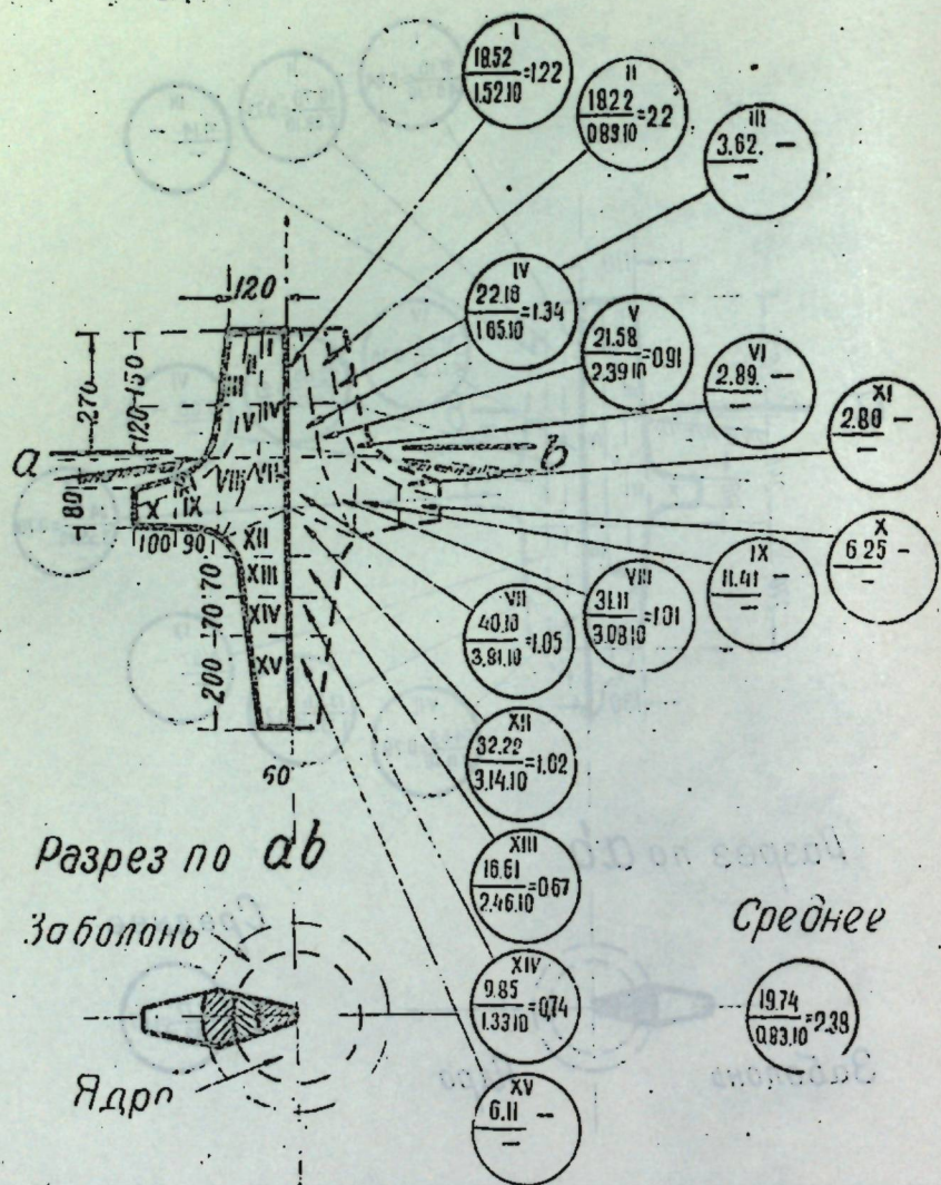
Схема распределения смолы и скипидара в сосновом пне. Образец № 3, взятый в Кестеньгском р-не, с. Кестеньга. Год рубки 1933. Год корчевки 1949.
