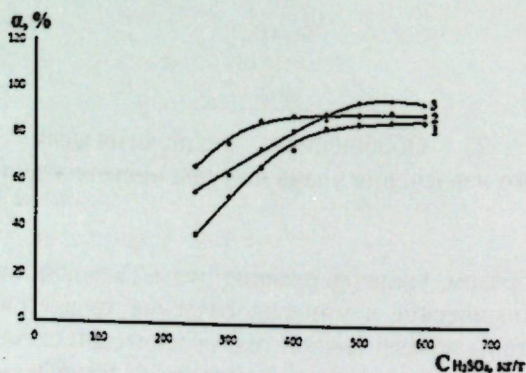
Рисунок 9. Сравнительная оценка степени выделения урана из различных руд урановых месторождений Таджикистана в зависимости от концентрации серной кислоты:
