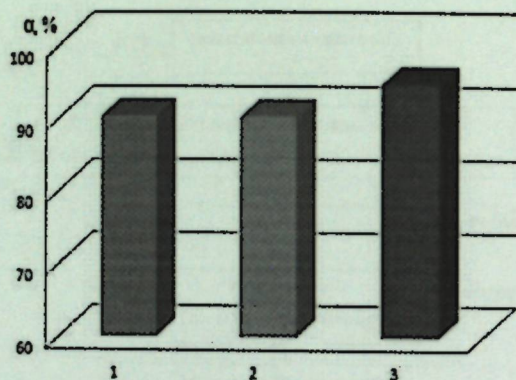
Рисунок 8. Сравнительная оценка степени извлечения урана из руды различных месторождений Таджикистана:
