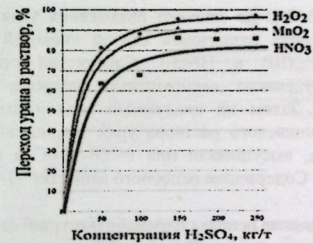
Рисунок 3. Влияние содержания H_2SO_4 на извлечение урана из руды при t=60^\circ C , T:Ж=1:2-5 , \tau=4 часа, C_{H_2O_2}=25 мл/л, C_{MnO_2}=50 кг/т и C_{HNO_3}=25 мл/л
