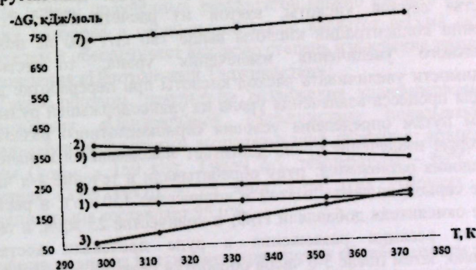
Рисунок 2. Зависимость изменения \Delta G от температуры разложения минералов, содержащихся в рудах месторождений "Западный Таджикистан" и "Центральный Таджикистан": 1) уранинит, 2) альбит, 3) пирит, 7) каолинит, 8) доломит, 9) сфен.
