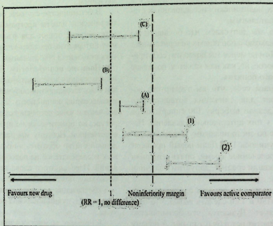
Рисунок 1. Графическая иллюстрация понятия noninferiority.
