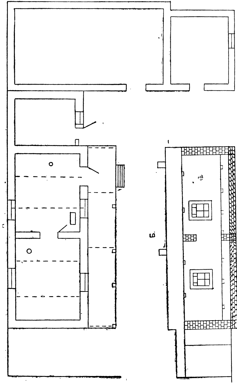
Рис. 34 План жилого дома из сырцового кирпича и с под ним. Сталина, с. Ак-Булун, Ново-Вознесен ворными постройками колхозника Шамирбекова. Колхоз ского района. А--план дома, Б--фасад дома.
