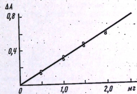
Рис. 3. Калибровочный график для определения алкалоидов, построенный по берберину бисульфату ΔA — разница оптической плотности между контролем и стандартом
