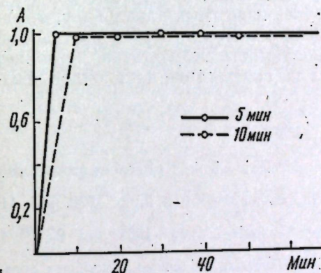
Рис. 2. Развитие интенсивности окраски раствора фосфорно-молибденовой кислоты 1 — нагревание 5 мин, 2 — нагревание 10 мин
