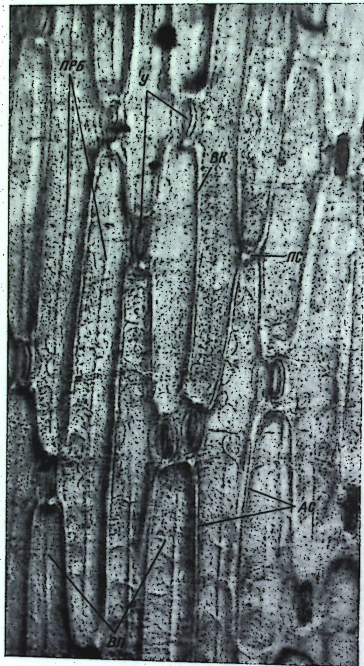
Рис. 3. Структура тангентальной поверхности периклиальной стенки клетки эпидермиса у A. gultschense ПРБ — продольные бороздки; ВК — выпуклость кутикулы над антиклинальными стенками клеток эпидермиса; АС — антиклинальные стенки клеток эпидермиса; ВП — восковые полоски, перпендикулярно направленные; У — устье
