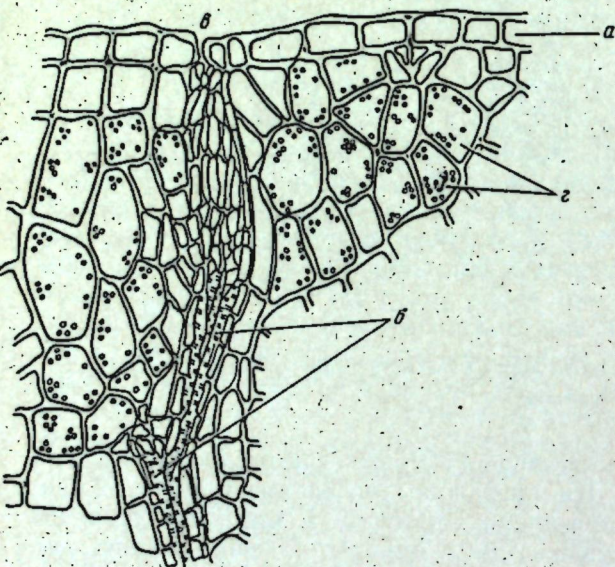
Рис. 4. Поперечный разрез листа Crassula perforata Thunb.
