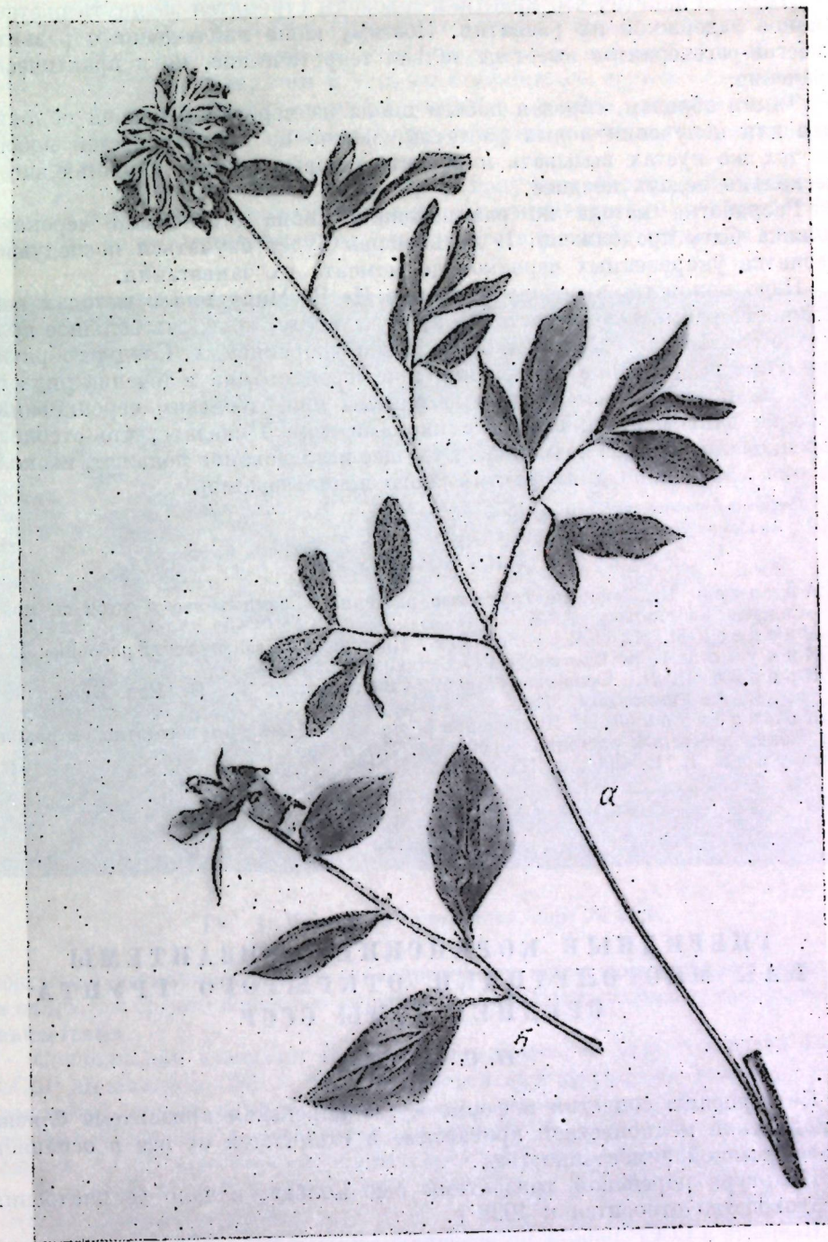
Рис. 4. Цветение побега-регенеранта (а). Внизу (б) показана верхушка основного побега с плодиками.
