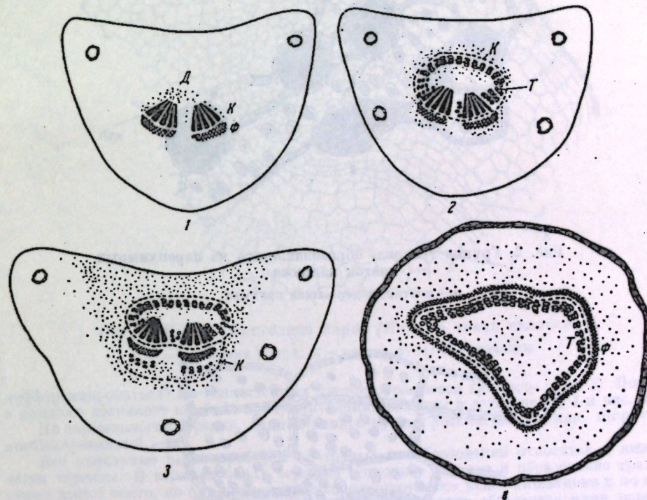
Рис. 1. Последовательные изменения в черешке листа Ginkgo biloba L.
