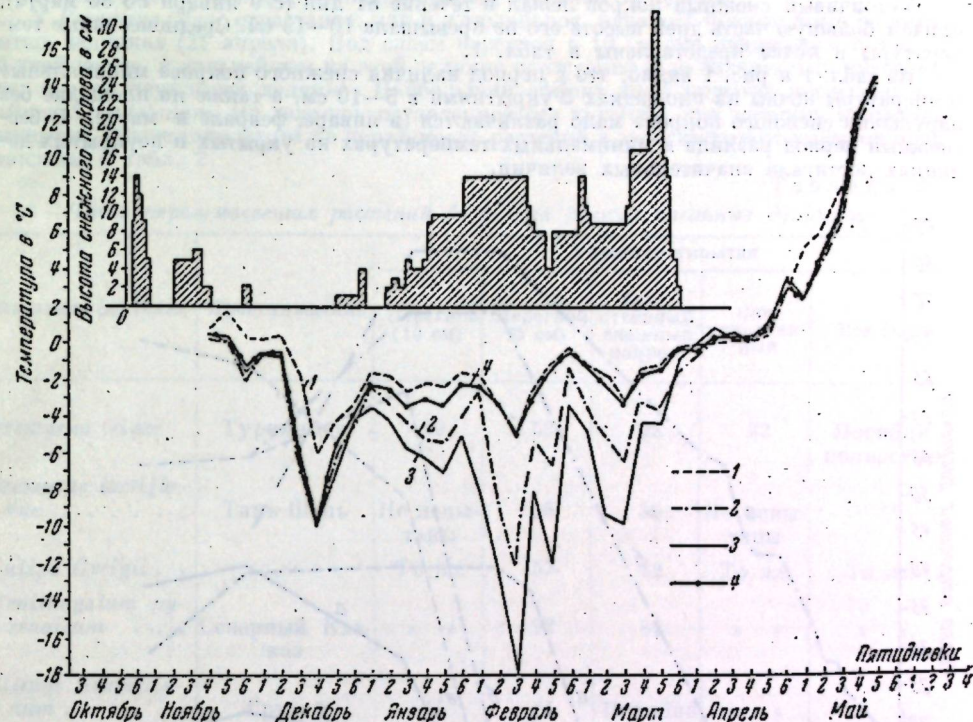
Рис. 1. Ход минимальной температуры в почве
