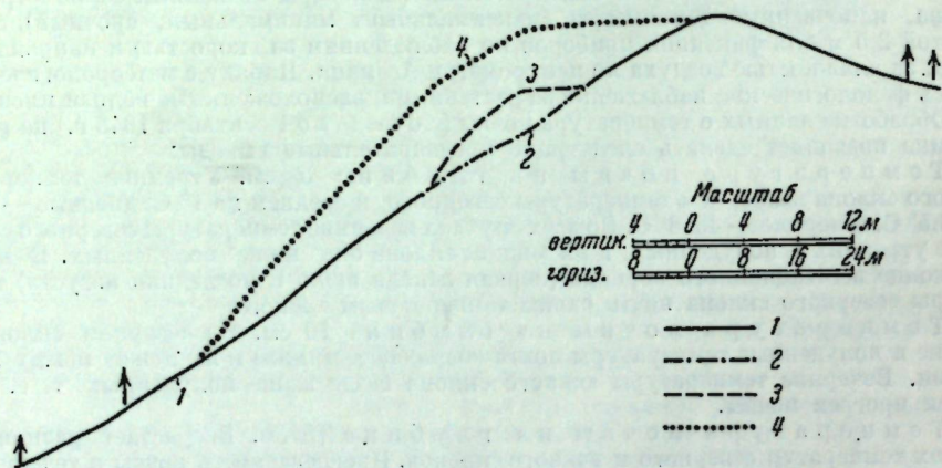
Рис. 1. Профиль седла перевала Кизи-Коницы
