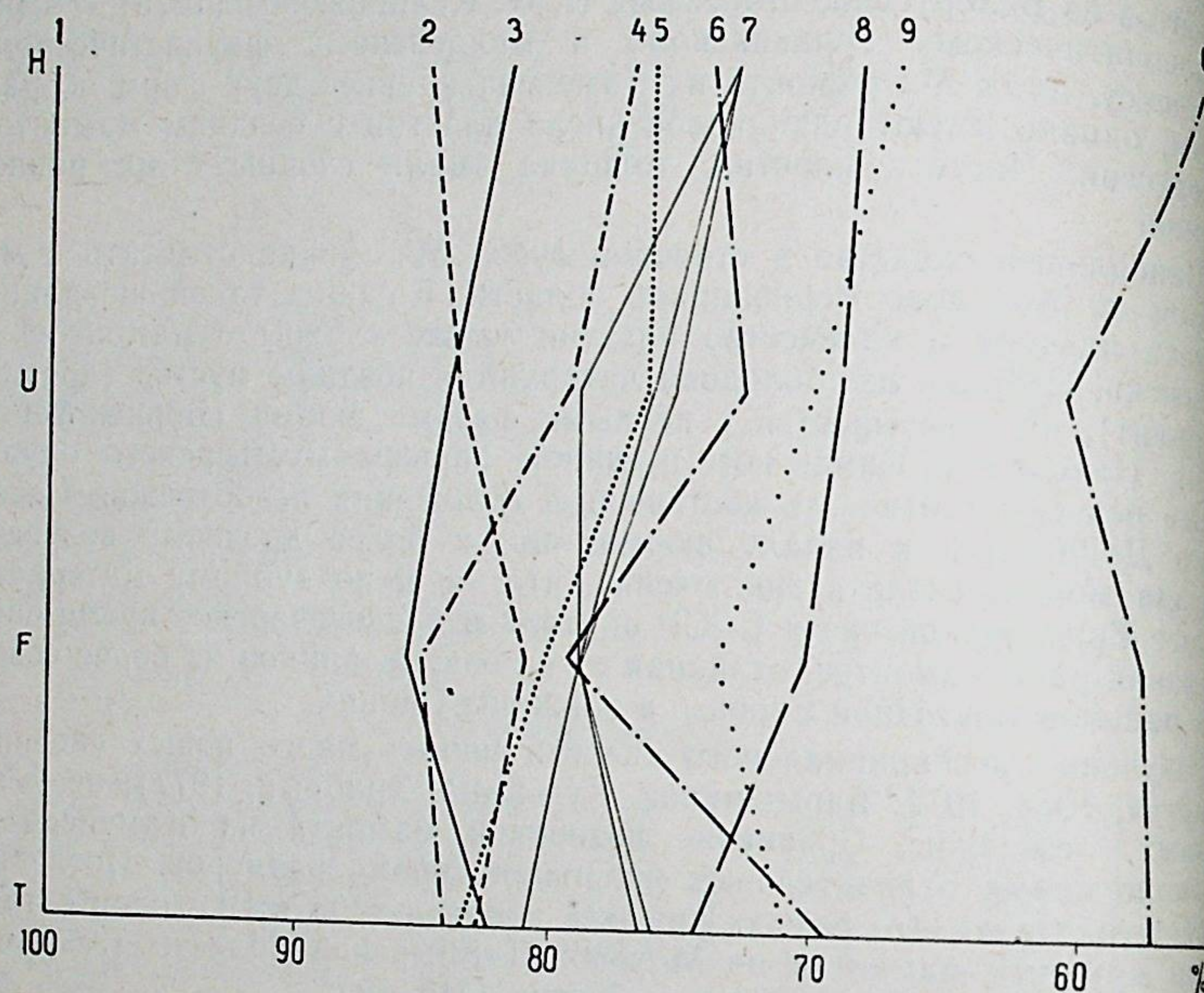
График уклонения длины трубчатых костей (H — Humerus, U — Ulna, F — Femur, T — Tibia) от принятых за 100% длины костей скелета Mammuthus primigenius fraasi из Штейнгейма (1) у слонов из местонахождений Борна (2), Пфеннерхаль (3), Новогеоргиевск (4), Лена (5), Берелех (6), Каменск (7), Березовка (8), Таймыр (9).
