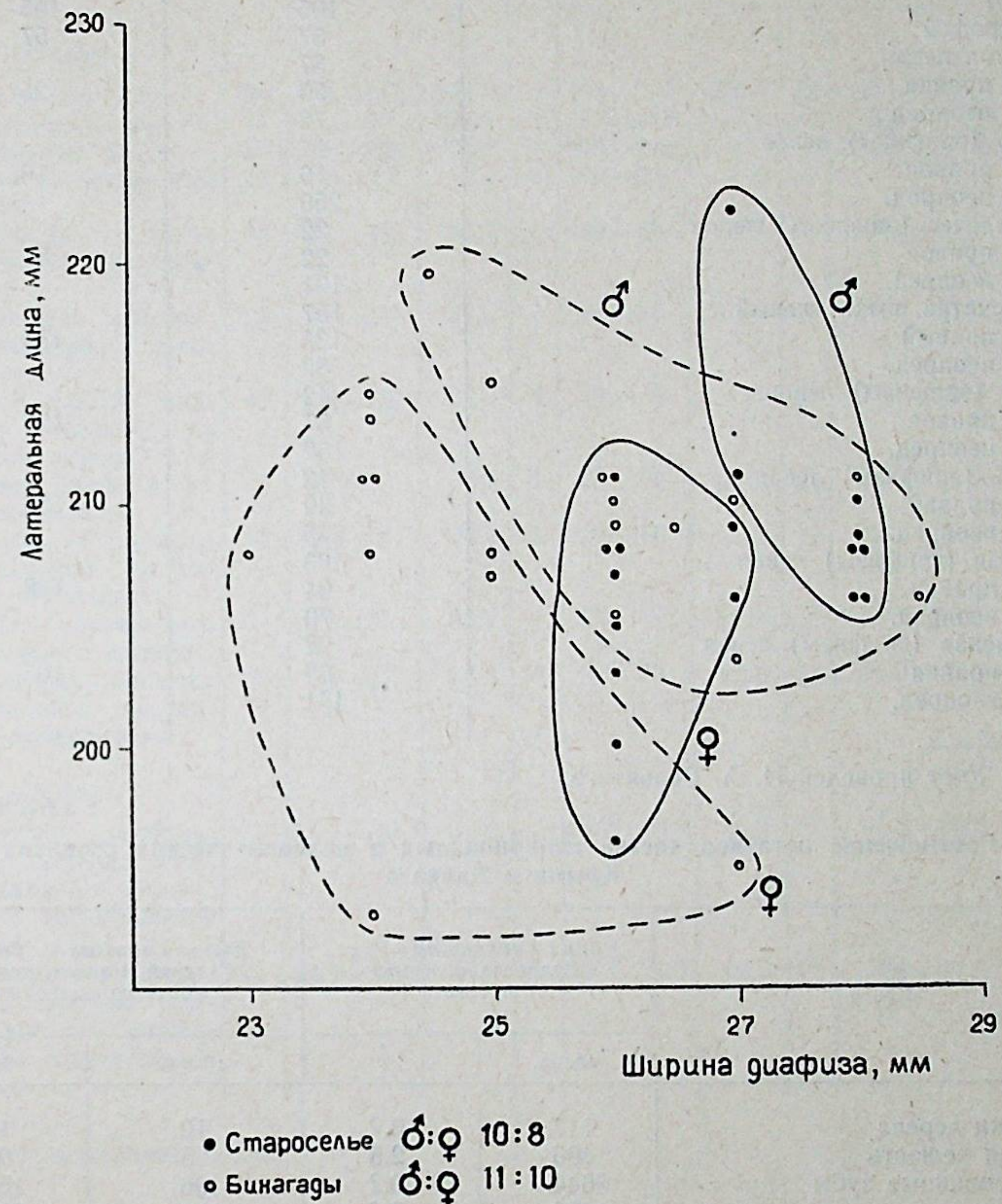
Рис. 5. Половая изменчивость пястных костей у плейстоценовых ослов Староселья и Бинагадов. Разделение по полу на основе пропорций
