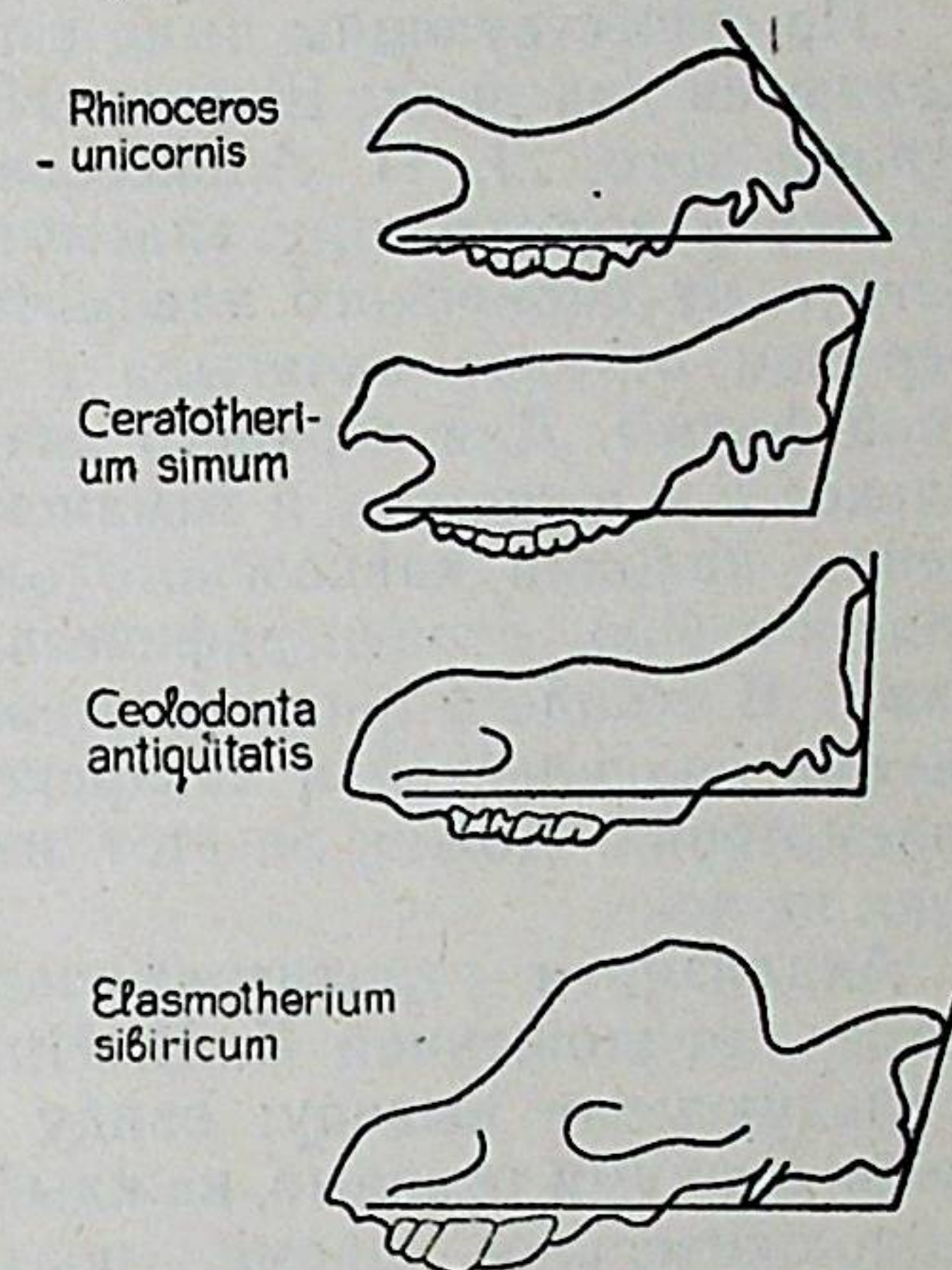
Рис. 2. Угол наклона плоскости затылочной части к линии основания черепа.
