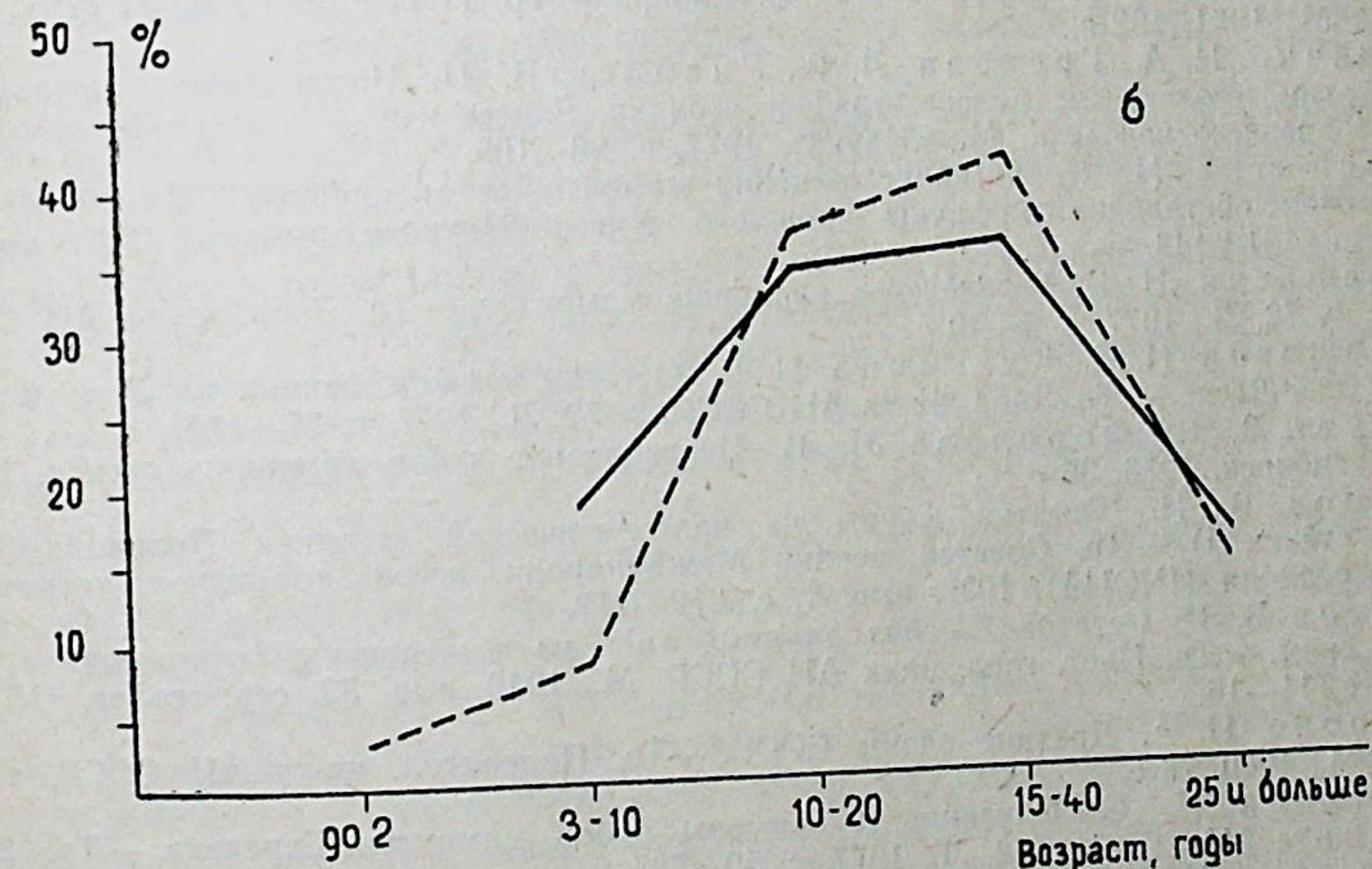
Рис. 4. Возрастной состав популяций мамонтов на основе анализа зубов: а — верхних, б — нижних, — Костенки, — — Берелех.
