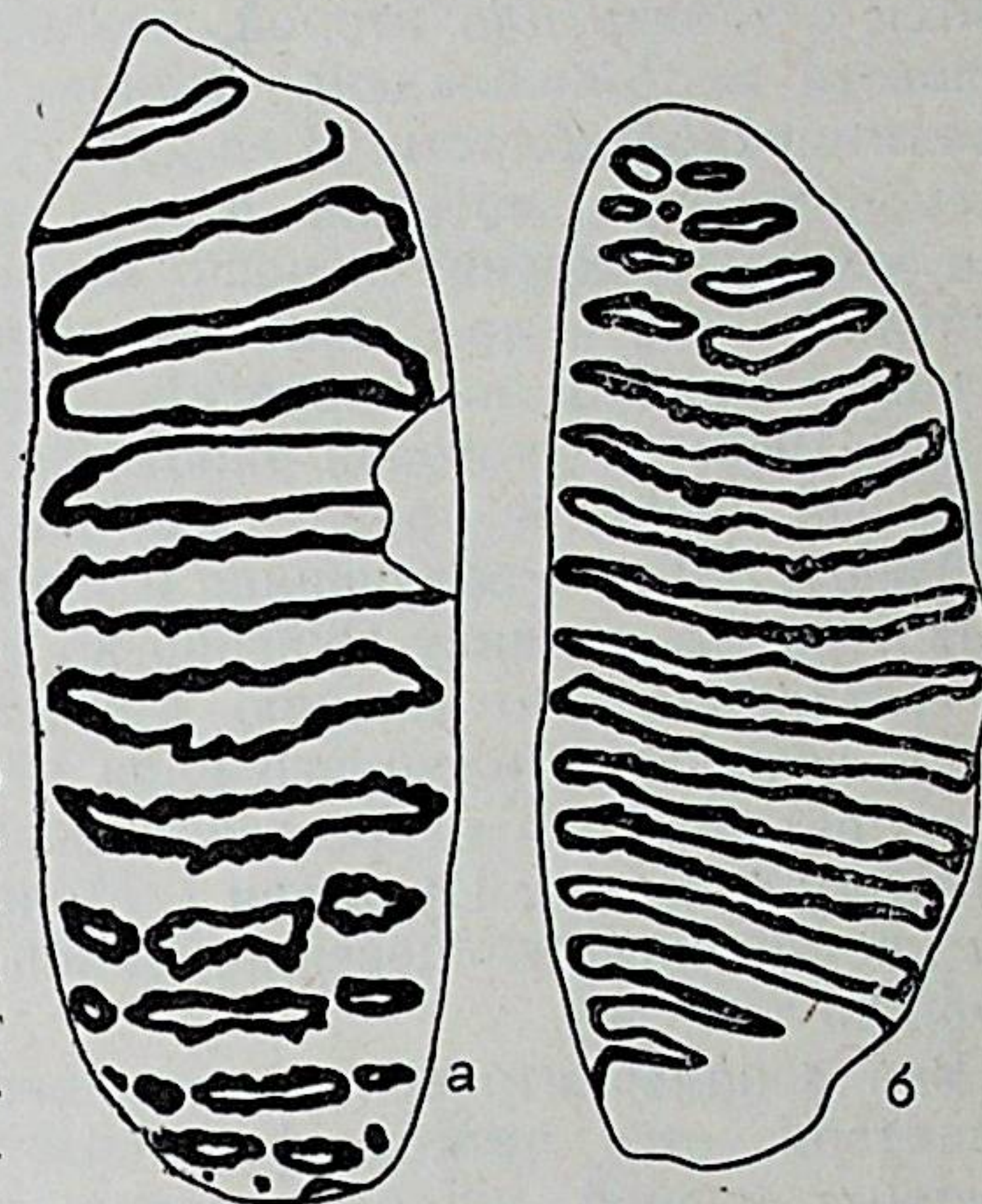
Эстампы жевательной поверхности зубов слонов из Шкурлатовского местонахождения (Воронежская область). М 1:2.
