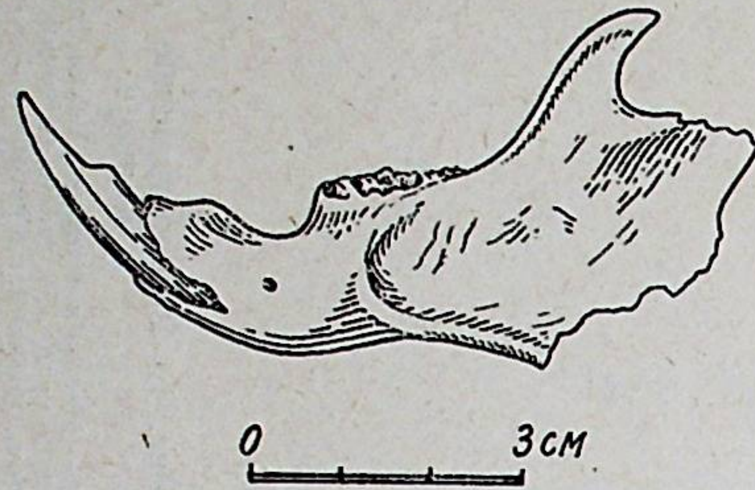
Рис. 2. Нижнечелюстная ветвь Marmota bobac paleocaucasica Baryshnikov subsp. nov. Голотип, колл. ЗИН АН СССР, № 31248.
