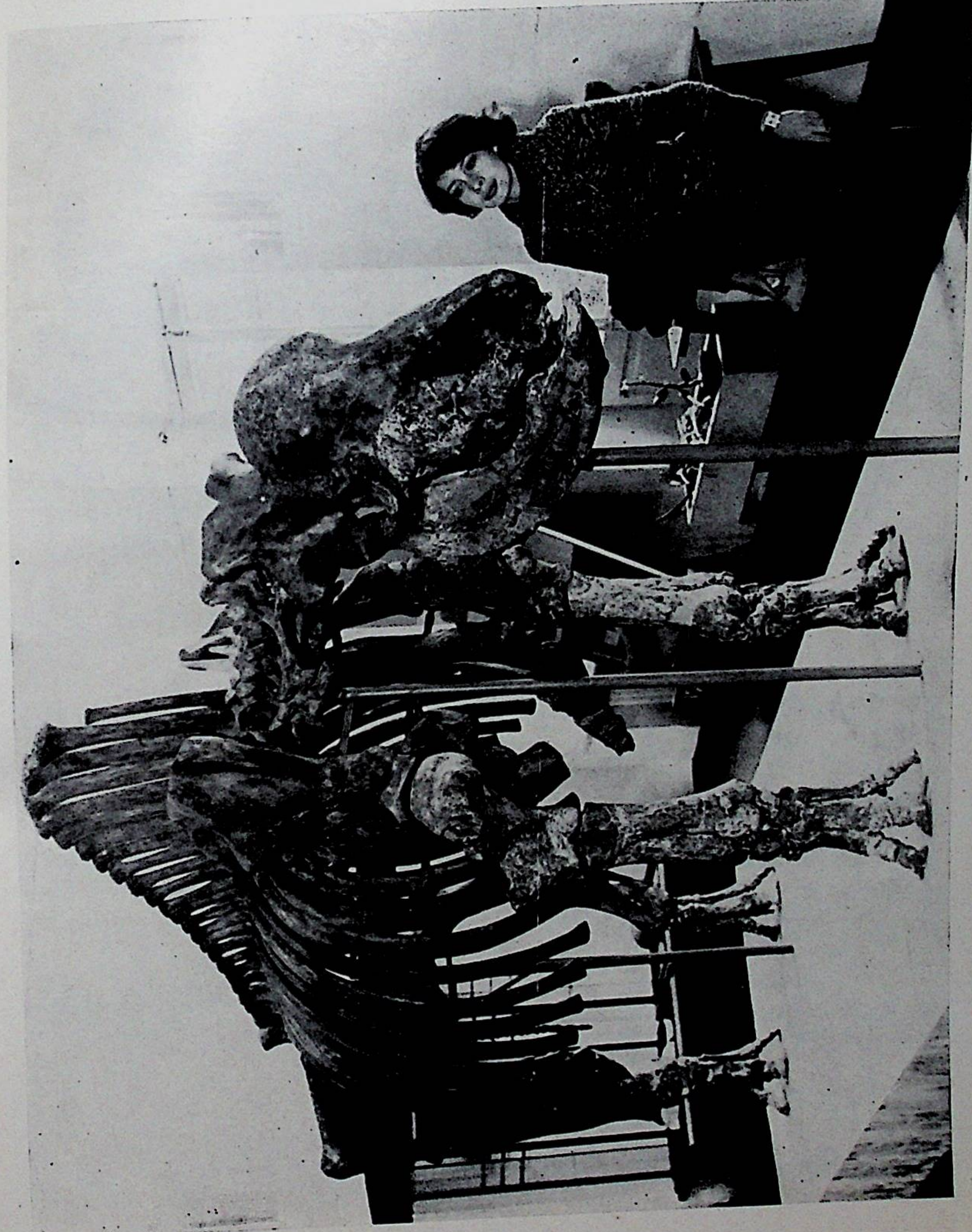
Рис. 1. Скелет эласмотерия Ставропольский краеведческий музей им. Г. К. Праве.
