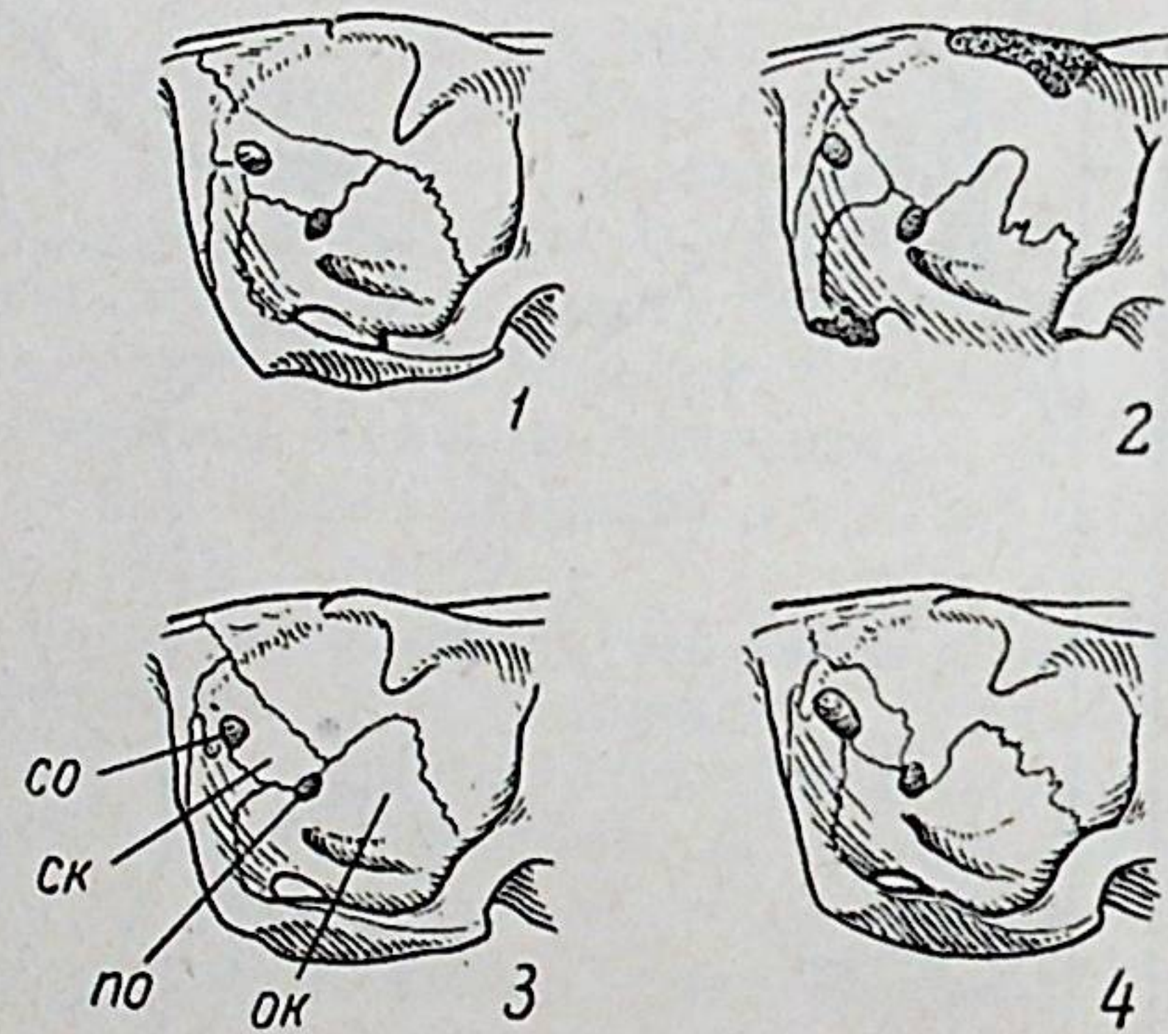
Рис. 3. Строение внутренней стенки орбиты у сурков.
