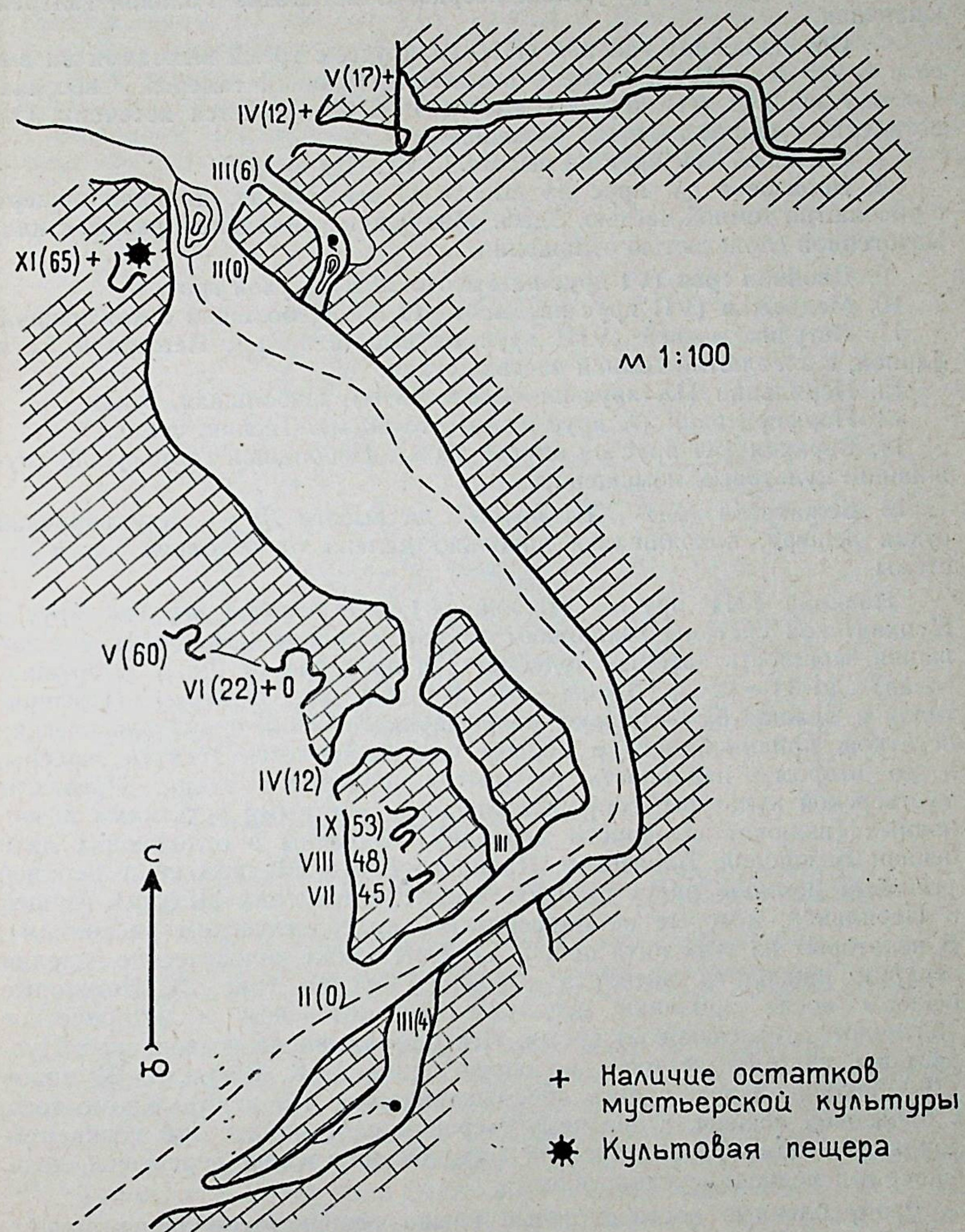
Рис. 1. План Цуцхватского пещерного комплекса.
