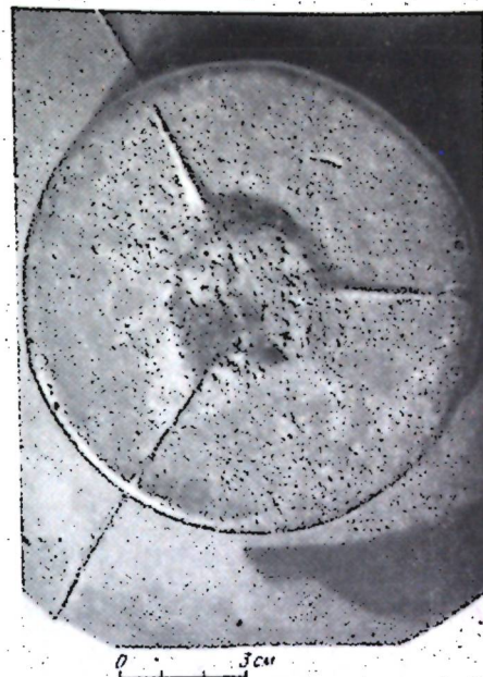
Рис. 3. Утолщение на дне сосуда — место подвода металла при отливке
