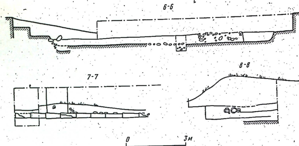
Рис. 2. Архитектурные разрезы
