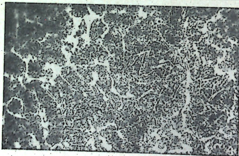
Рис. 2. Образцы микроструктур чугуна из Тоджи
