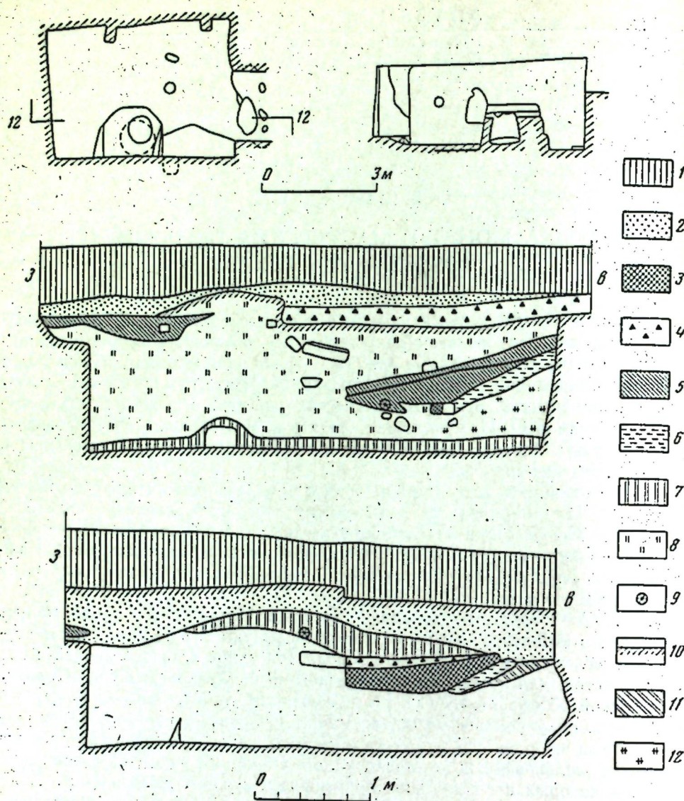
Рис. 1. Пенджикент. Объект XVI. План и разрезы мастерской (помещение 72)
