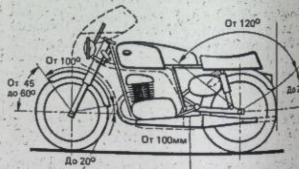
Испытательный мотоцикл.
