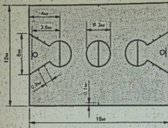
Площадка для игры в мини-баскетбол.
