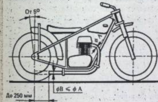
Мотоцикл для спидвея.
