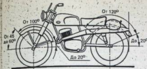
Мотоцикл для гонок по шоссе.
