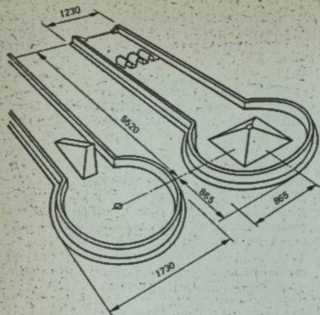
Площадки для игры в мини-гольф с трамплином и плоской пирамидой.
