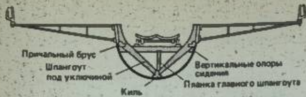
Треугольная конструкция, препятствующая «закручиванию» судна.
