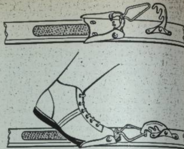
Крепления для лыжных гонок системы «Роттафелла».
