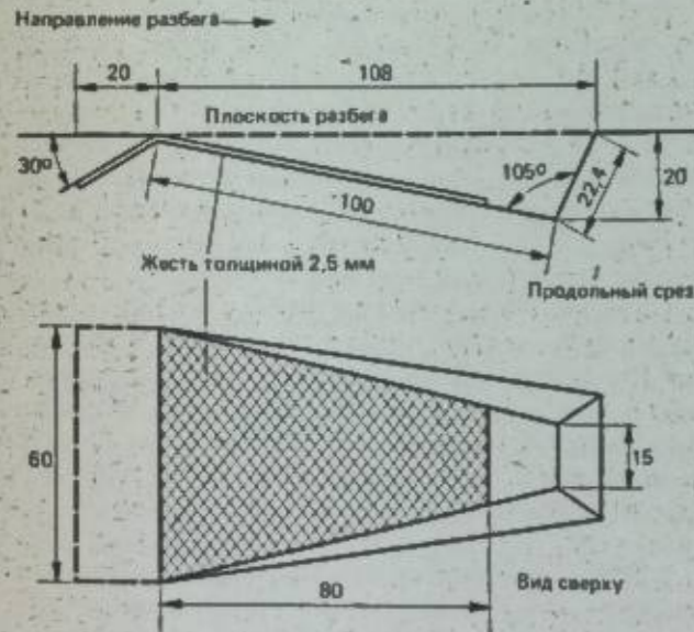
Ящик для упора шеста.
