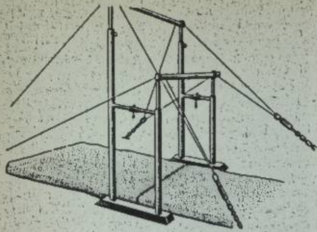
Разновысокие брусья системы Ройтера.
