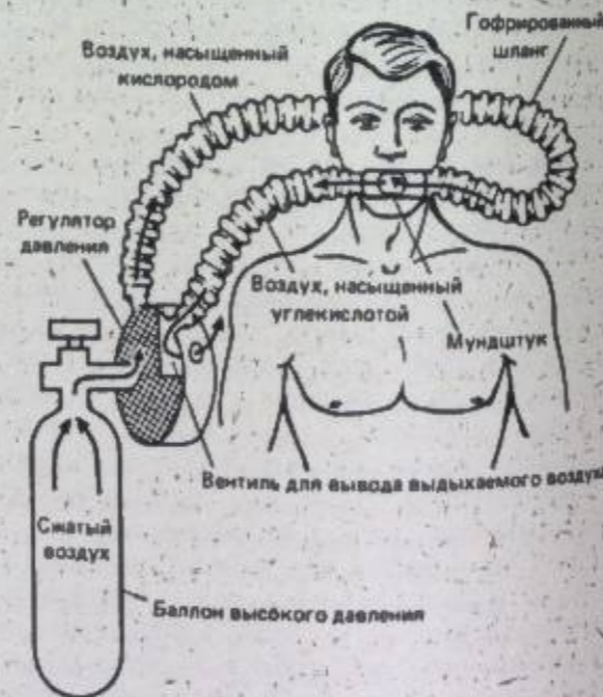
Аппарат со сжатым воздухом и принцип его действия.
