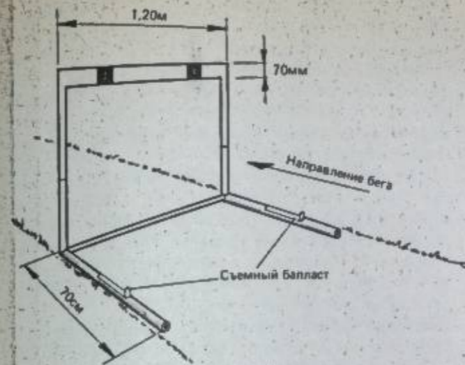
Барьер из стальной трубки.
