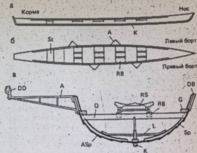
Названия частей судна: а) вид сбоку; б) вид сверху; в) поперечный разрез. А — стержень распашной uključины; Asp — шпангоут под uključиной; DB — фальшборт; DD — вращающаяся uključина; G — причальный брус; K — киль; L — полки; Q — планка главного шпангоута; RB — полозья; RS — подвижное сиденье; Sp — шпангоут; St — сиденье для рулевого.
