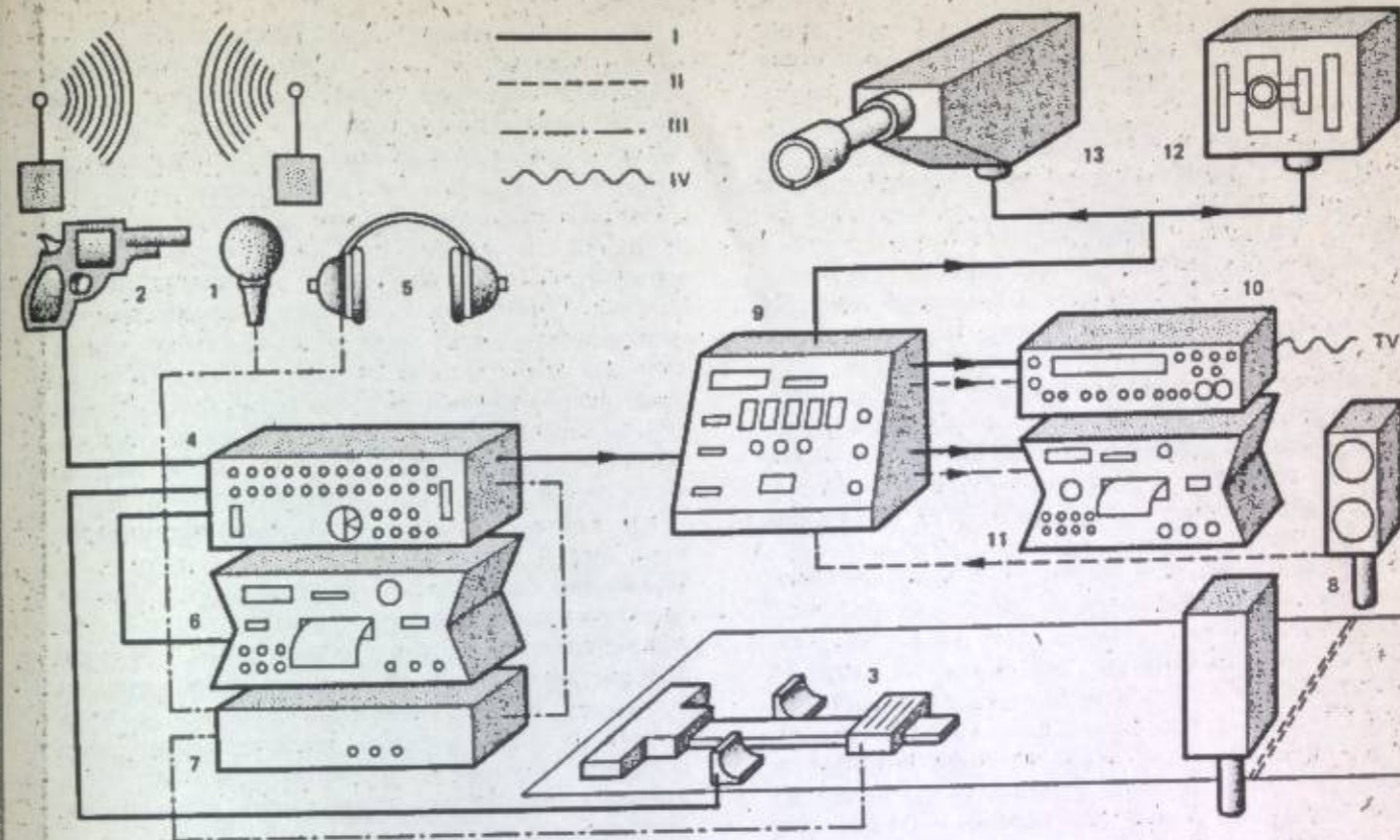
Хронометрирование: электронное хронометрирование в легкой атлетике (по системе Юнгханса): 1. стартовая команда через микрофон; 2. стартовый сигнал стартовым пистолетом, отсчет времени начат; 3. стартовый прибор с вмонтированным громкоговорителем и нажимным контактом (импульс от нажатия на стартовые колодки передается к «стартовому ассистенту»); 4. «стартовый ассистент» для измерения времени реакции, подачи сигнала о фальстарте и передачи стартового импульса через 9 на 10-13; 5. наушники; 6. устройство, печатающее данные о времени реакции; 7. усилитель; 8. двойной световой затвор, стоп-импульс передается через 9 на 10 и 11; 9. пульт управления; 10. «каунтер 7202» (хронометр с кварцевой стабилизацией) для передачи информации на табло и на телевидение; 11. устройство, печатающее результаты хронометрирования; 12. «Пола-Хрон», выдает позитивы фотофиниша; 13. «Фото-Хрон», выдает последовательную серию негативов фотофиниша; I-стартовый импульс от пистолета; II-стоп-импульс от светового затвора; III-громкоговоритель; IV-передача информации.
