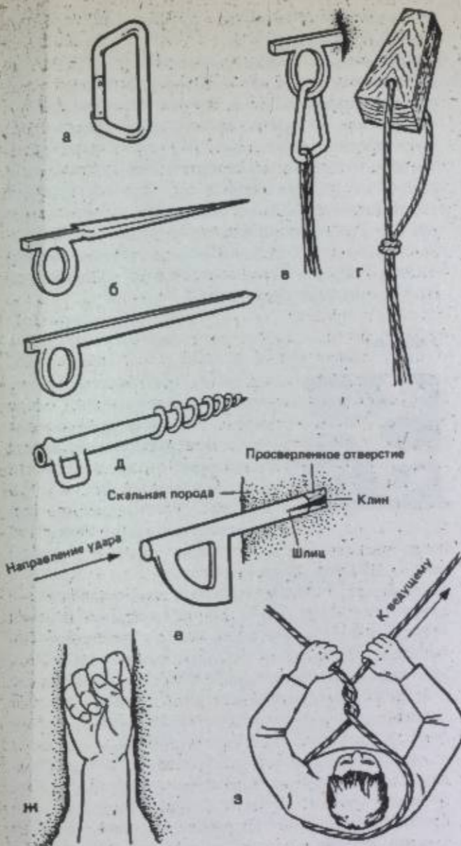
а) крюк с карабинной защелкой; б) и в) скальные крюки; г) деревянный клин; д) трубчатый виэт для бурения льда; е) действие бурового крюка (надписи по часовой стрелке: направление удара; скальная порода; просверленное отверстие; клин; шлиц); ж) техника введения руки в щель; з) страховка двойным перекрещиванием каната.
