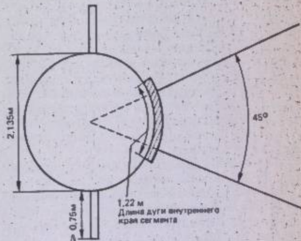
Сектор для толкания ядра.
