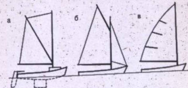
Виды оснащения судов: а) шпрюйт; б) шлюп; в) кэт.
