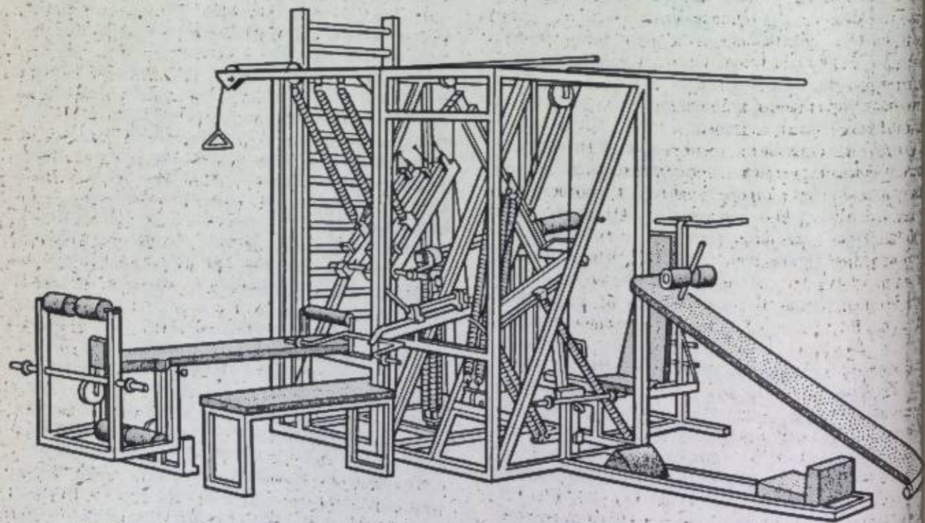
Снаряд для силовой тренировки с пружинящими сопротивлениями, рассчитанный на работу «станциями».
