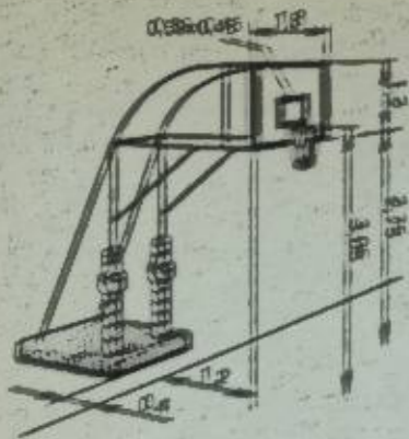
Баскетбольная стойка со щитом и корзиной.
