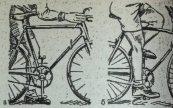
Подгонка велосипеда: а) расстояние между концами седла и рулем; б) высота седла.
