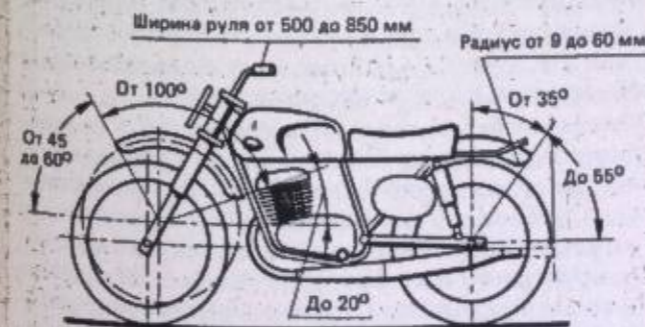
Мотоцикл для кросса.
