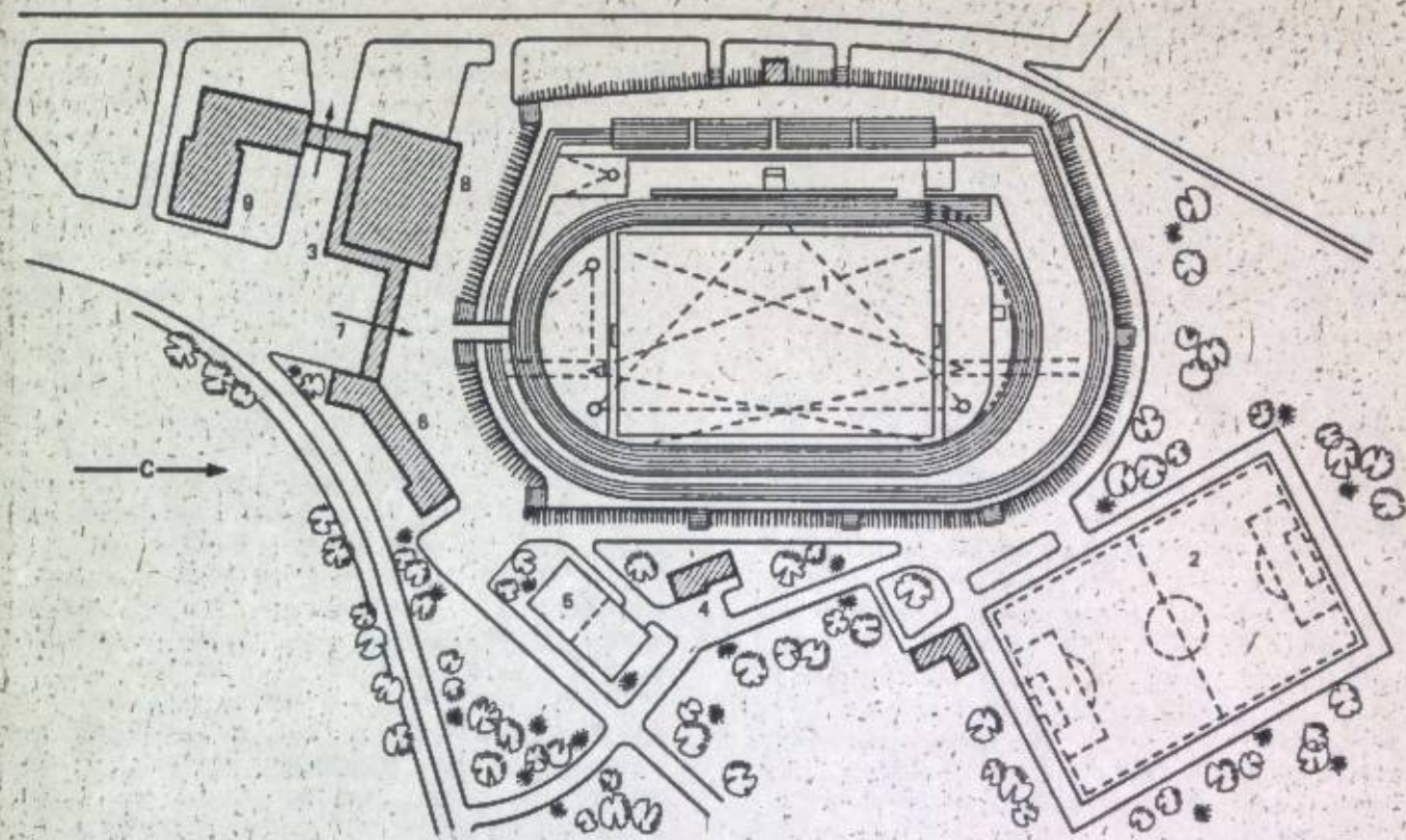
Спортивный комплекс (пример использования): 1. большая спортивная арена; 2. малая спортивная арена; 3. раздевалки; 4. помещение для охраны; 5. площадка для фаустбола; 6. кегельбан; 7. проходная; 8. спортивный зал; 9. столовая.
