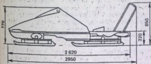
Бобслей-двойка (размеры в мм).
