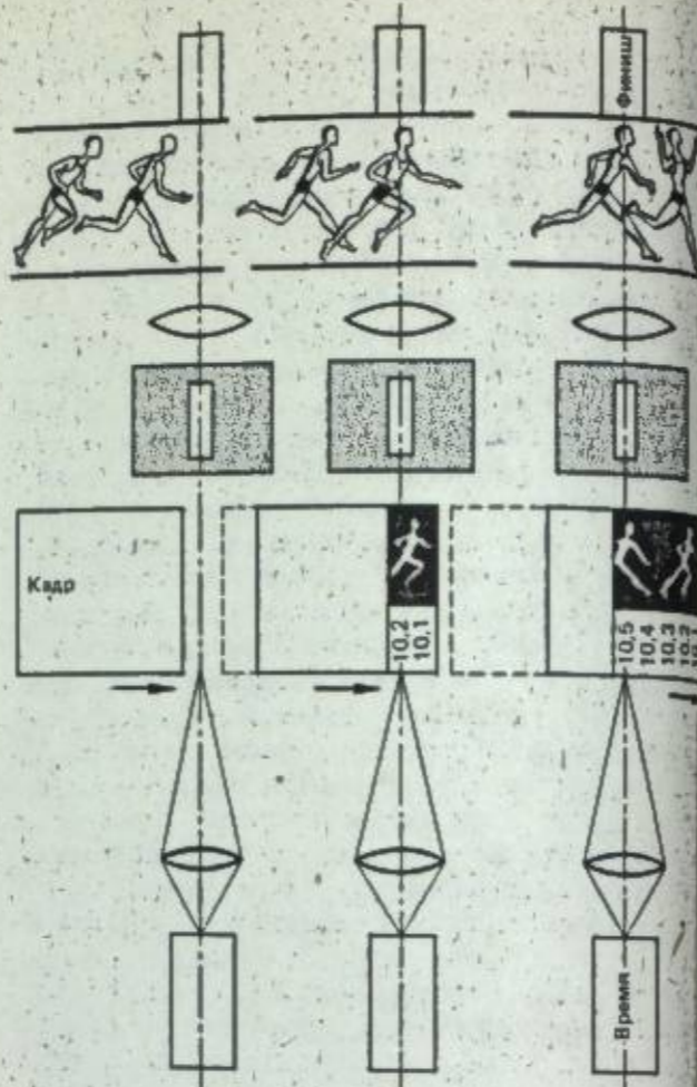
Схема работы фотофиниша.
