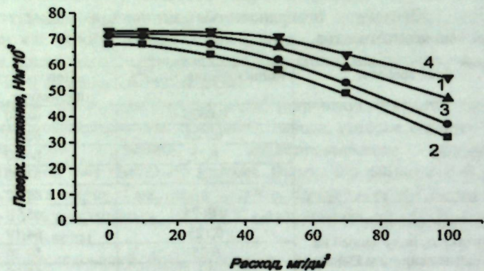
Рисунок 1 - Зависимость поверхностного натяжения (σ) водных растворов аэрофлотов от концентрации: 1 - смесь №1; 2 - бутиловый аэрофлот; 3 - смесь №3; 4 - смесь №2.
