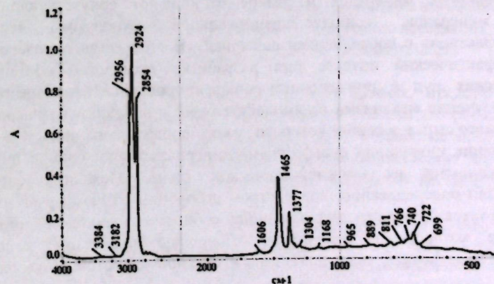
Рисунок 3 - Инфракрасный спектр пробы дизельного топлива.
