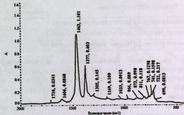
Рисунок 2 - Инфракрасный спектр пробы нефти Кумкольского месторождения.
