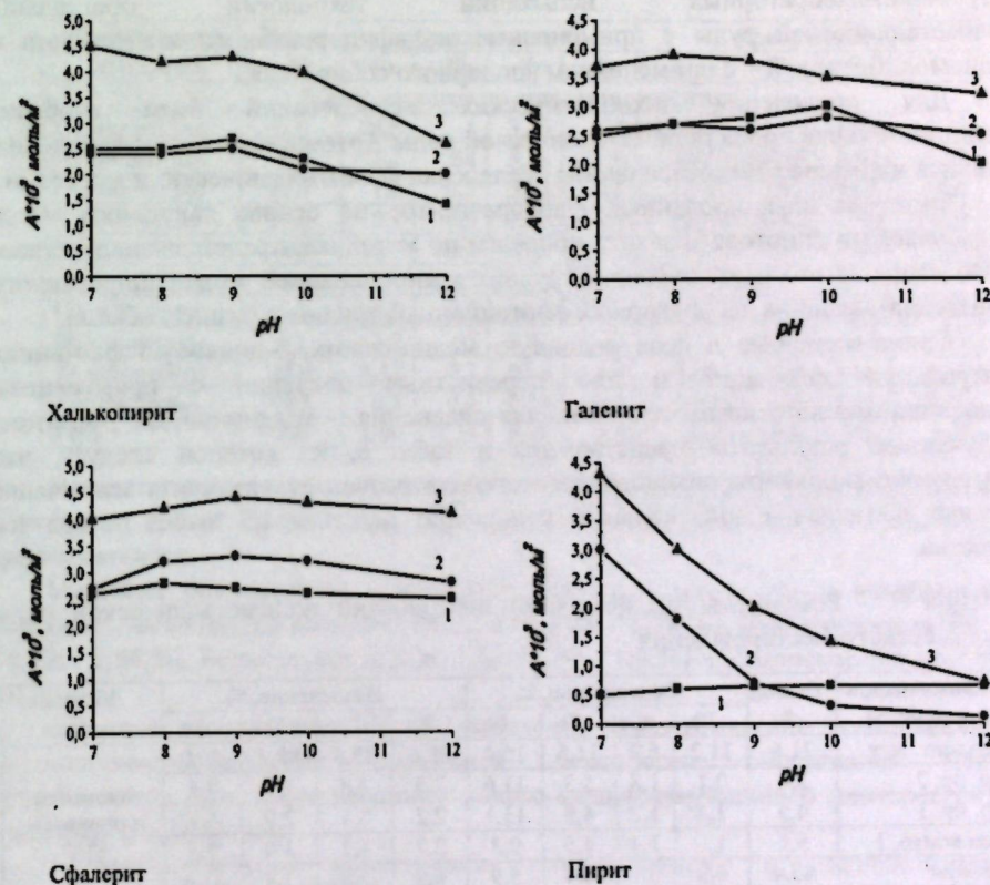
Рисунок 4 - Изменение концентрации композиционного аэрофлота на сорбированных мономинералах при разных pH в процессе десорбции: водой (1); этанолом (2); смесью гексана с соляной кислотой (3).
