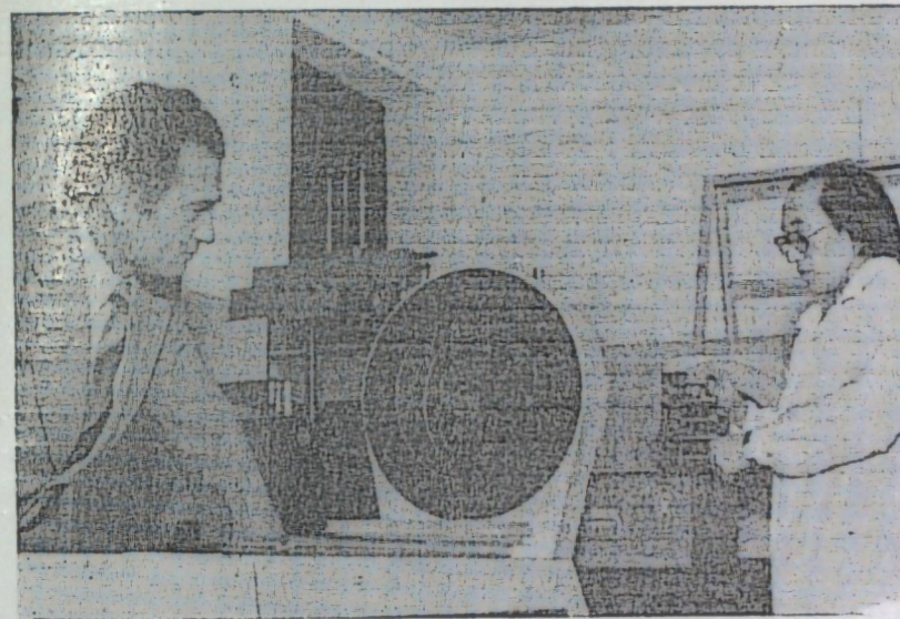
Исследование напряженного состояния массивов горных пород с помощью фотоупругих моделей.
