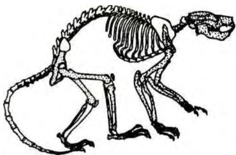
Рис. 10. Плезиадапис
