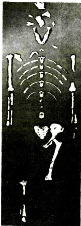
Рис. 21. Скелет «Люси»
