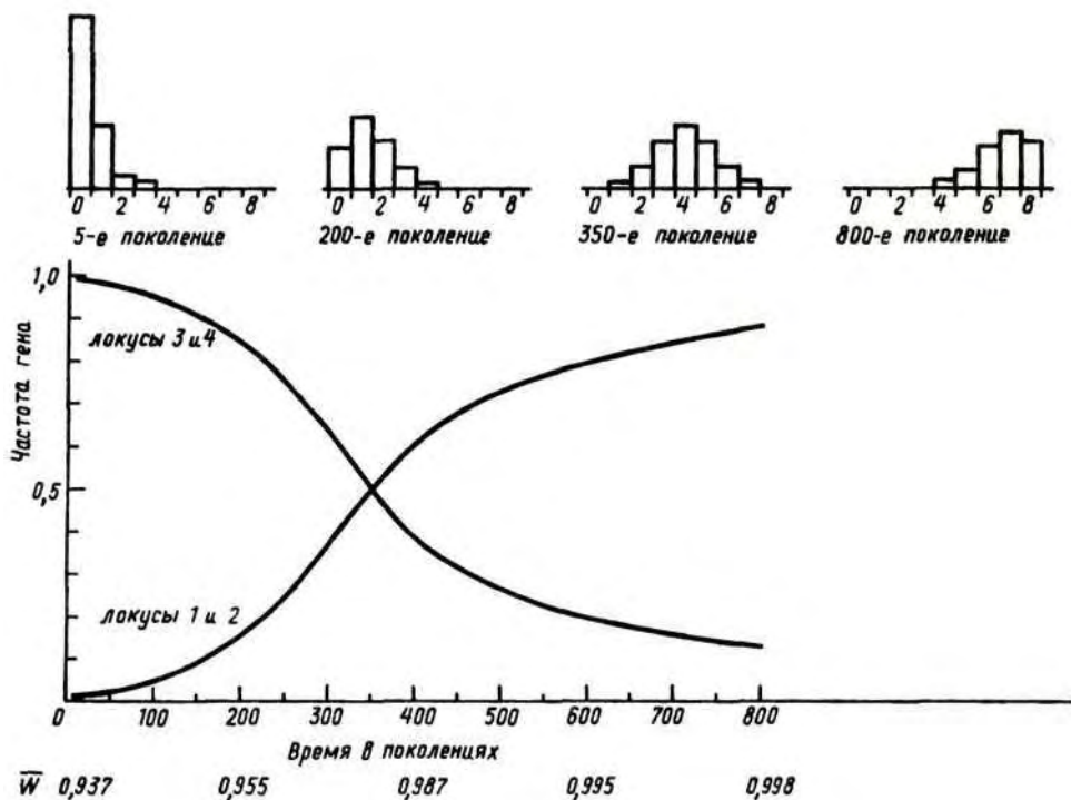
Рис. 112. Изменение частот аллелей и распределение фенотипов в модельном эксперименте эволюции темного цвета кожи при отсутствии доминантности с другими значениями поиспособленности (Livinstone. 1969)
