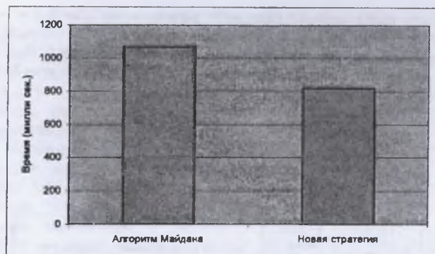
Рис. 2. Время выполнения
