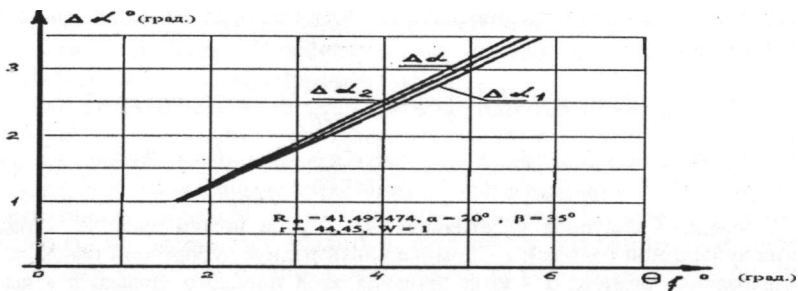
Рис.2. График отклонения угла профиля \Delta\alpha в зависимости от угла ножки \theta_f .
