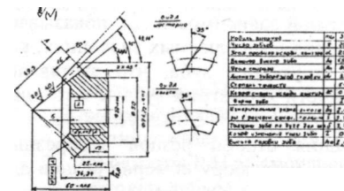
Рис.8. Коническая передача с круговыми зубьями
