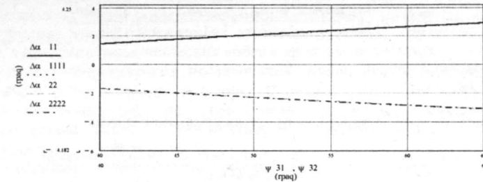
Рис.7. Графики \Delta\alpha_{11} и \Delta\alpha_{22} - кривые теоретических исследований отклонений угла профиля по вогнутой и выпуклой стороне в диапазоне профилирования эвольвенты зуба, графики \Delta\alpha_{1111} и \Delta\alpha_{2222} - кривые моделирования настройки модификатора обкатки для получения расчетных отклонений угла профиля по вогнутой и выпуклой стороне зуба
