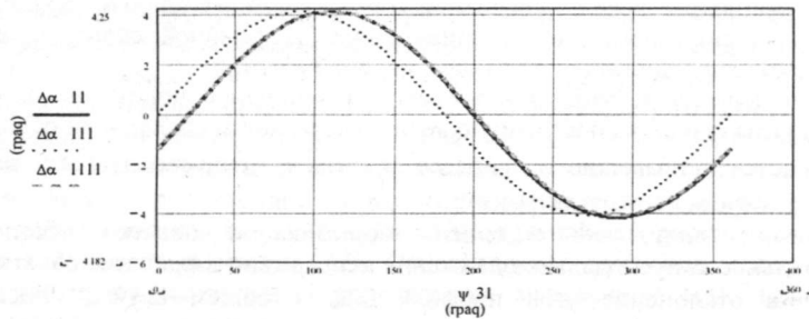
Рис.6. Сравнительные графики отклонений угла профиля по вогнутой стороне зуба, описываемых различными зависимостями: \Delta\alpha_{11} - формула (7), \Delta\alpha_{111} - формула (8), \Delta\alpha_{1111} - формула (9).
