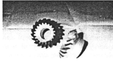
Рис.10. Процесс обработки конических колес.
