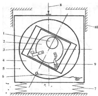
Рис.17. Конструктивная схема синусного МПС
