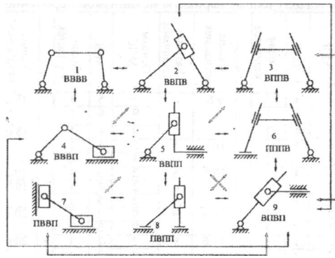
Рис.3. 1-шарнирно-четырёхзвенный механизм, 2-кулисный механизм, 3-механизм Ольдгейма, 4-кривошипно-ползунный механизм, 5-синусный механизм, 6-8-механизмы Добровольского с вращательной развязкой, 7- механизм эллипсографа, 9- тангенсный механизм.
