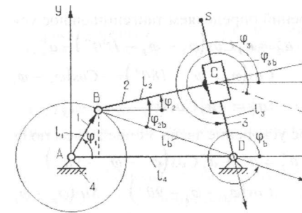
Рис. 10. Расчетная схема кулисного механизма, имеющего смещение камня
