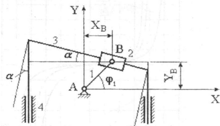
Рис.18. Кинематическая схема синусного механизма
