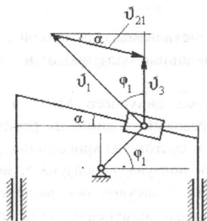
Рис. 19. План скоростей.
