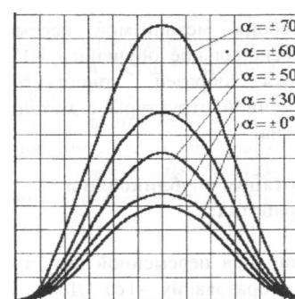
Рис.21. График зависимости перемещения ползуна от угла поворота кривошипа
