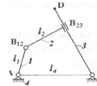
Рис.5. Схема кулисного механизма
