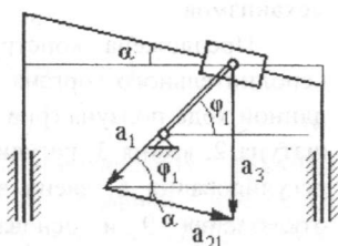
Рис.20. План ускорений.
