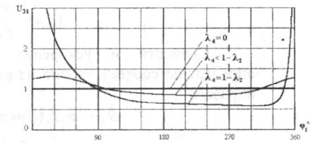
Рис. 16. Зависимость передаточного отношения U_{31} от угла \varphi_1 при \lambda_2 = 0,5 .
