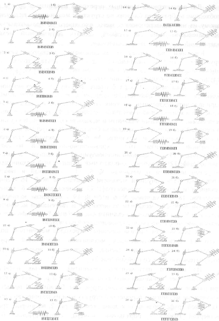
Рис. 2. Полученные схемы механизмов переменной структуры
