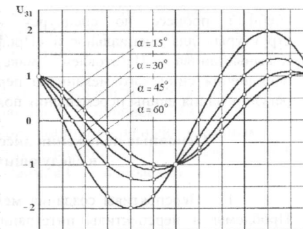
Рис.22. График зависимости передаточного отношения ползуна от угла поворота кривошипа
