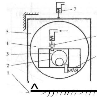
Рис. 9. Конструктивная схема кривошипно-кулисного МПС.
