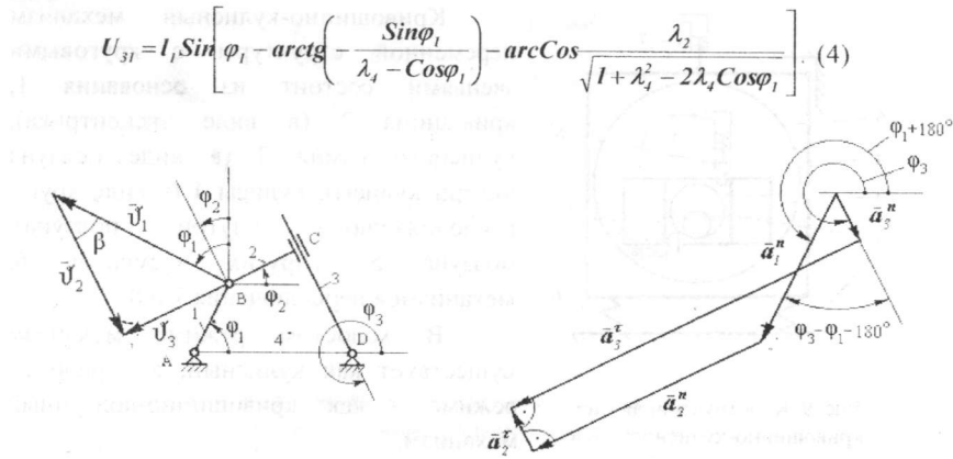
Рис. 11. План скоростей.
