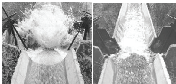
Фото 5 (а, б). Водораспределительные сооружения на внутрихозяйственных лотковых каналах параболического сечения: а – водораспределитель без козырька; б – водораспределитель с козырьком
