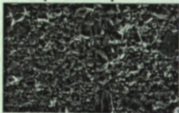
Рис. 2.1. Изображение электронного микроскопа частиц галенитсодержащих концентратов месторождения Кони Мансур (Республика Таджикистан).
