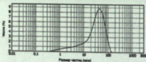
Рис. 2.2. Распределение размеров частиц галенитсодержащих концентратов месторождения Кони Мансур (Республика Таджикистан).
