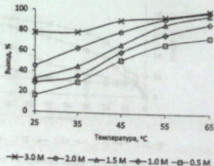
Рис. 3.1.3. Влияние температуры на выход свинца при разных концентрациях кислоты.
