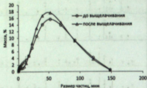
Рис. 3.4.1. Распределение размеров частиц галенитсодержащего концентрата до и после выщелачивания.
