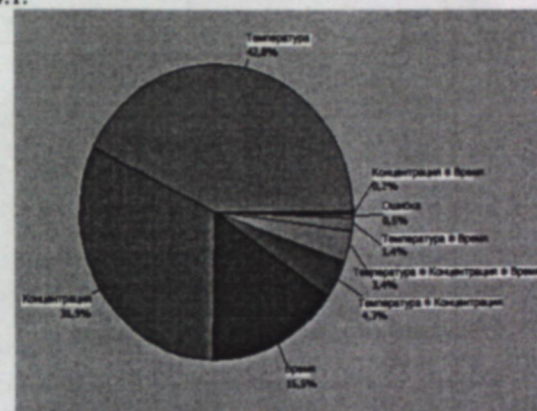
Рис. 4.1. Круговая диаграмма значений выхода Pb из галенитсодержащего концентрата месторождения Кони Мансур.
