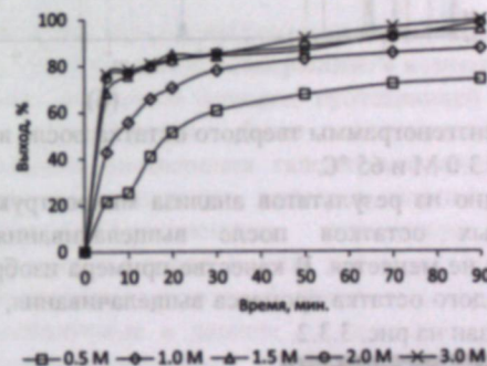
Рис. 3.2.1. Зависимость степени извлечения свинца от концентрации кислоты и времени для галенитсодержащих концентратов месторождения Кони Мансур при 65 °C.
