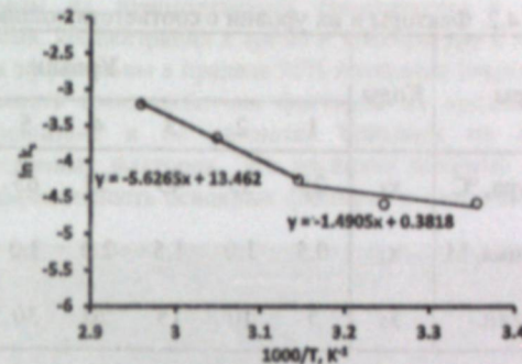
Рис. 3.4.3. Зависимость константы скорости реакции от температуры для галенитсодержащего концентрата.
