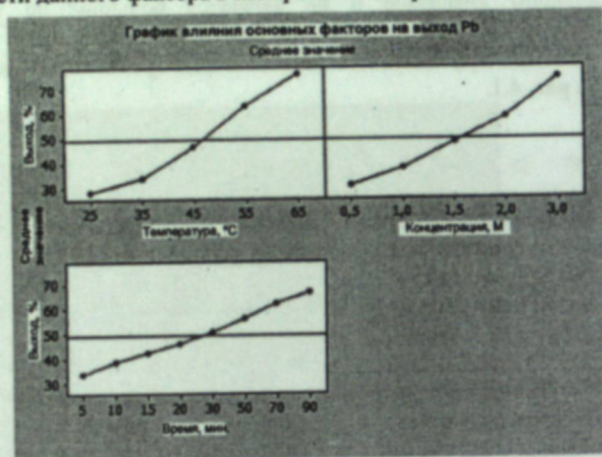
Рис. 4.2. Влияние основных факторов на выход Pb для галенитсодержащих концентратов месторождения Кони Мансур.
