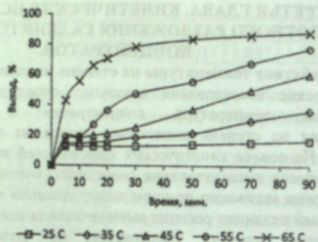
Рис. 3.1.2. Зависимость степени извлечения свинца от температуры и времени при концентрации кислоты 1.0 М.
