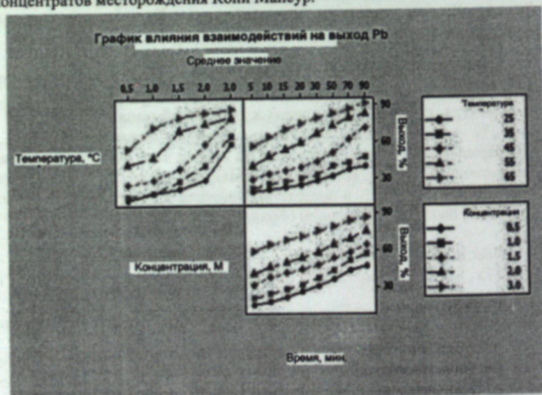
Рис. 4.3. Влияние взаимодействий факторов на выход Pb для галенитсодержащих концентратов месторождения Кони Мансур (республика Таджикистан).
