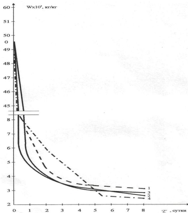
Рис.9. Изменение содержания влаги в образцах типичного серозема с добавками гуминовых удобрений и стимулятора роста растений при высушивании над безводным гипсом: 1– исходная почва +5% гуматов аммония; 2– исходная почва +0,5% гумата натрия; 3– исходная почва +0,5% гумат – силикатный композит; 4– исходная почва.
