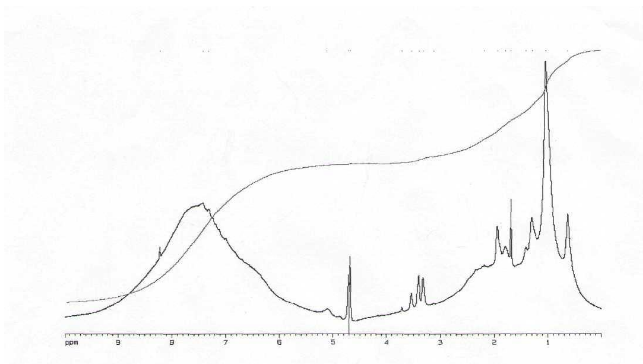
Рис.3. ^1\text{H} -ЯМР спектр ГК (уголь Кара-Кече).
