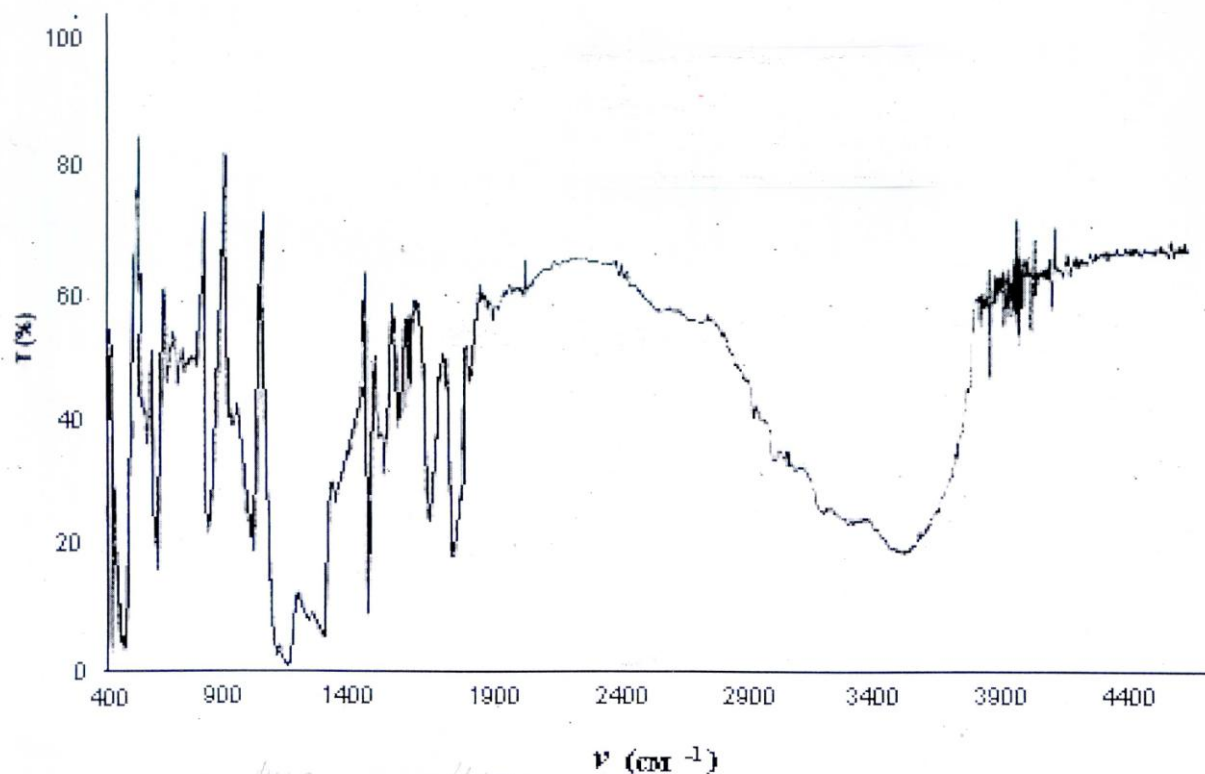
Рис.4. Инфракрасные спектры гуминовых удобрений (гумофос).
