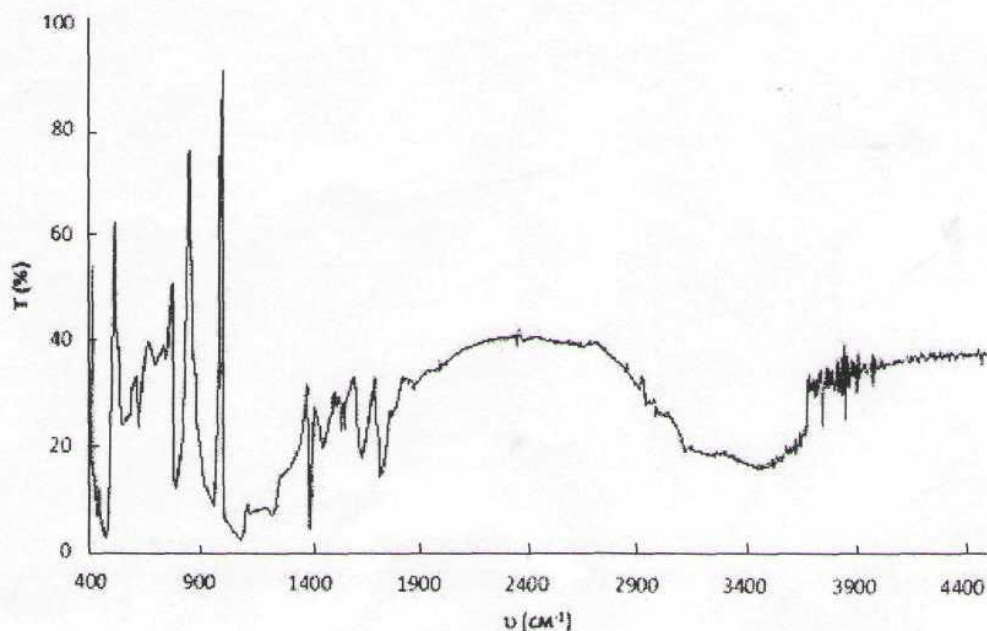
Рис.5. ИК - спектры гумат – силикатного композита.
