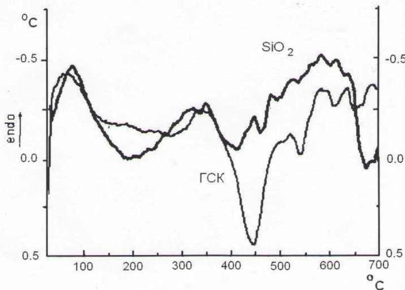
Рис.7. DTA кривые для \text{SiO}_2 и ГСК ( атмосфера \text{O}_2 ).
