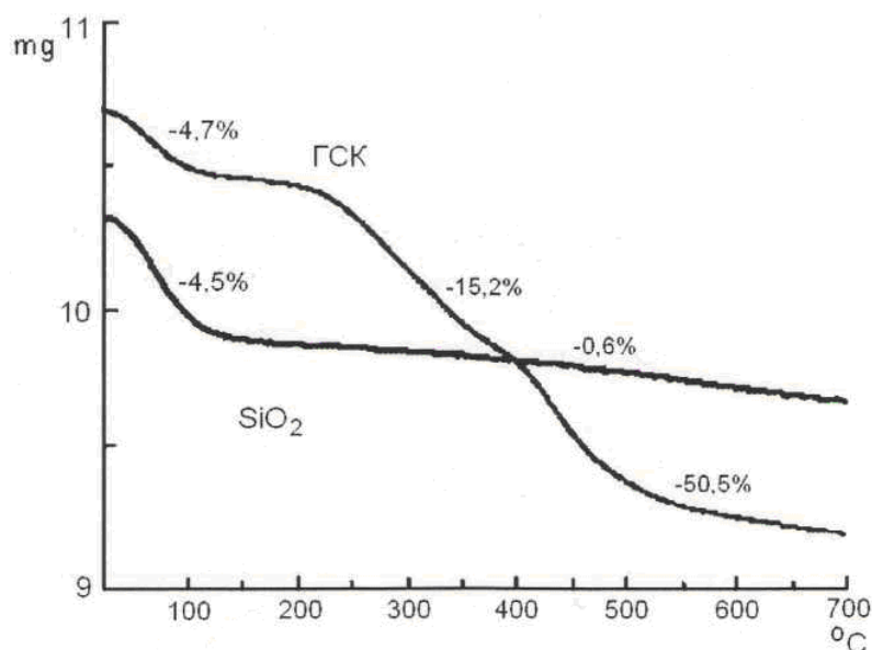
Рис.6. TG кривые для SiO 2 и ГСК ( атмосфера O 2 ).
