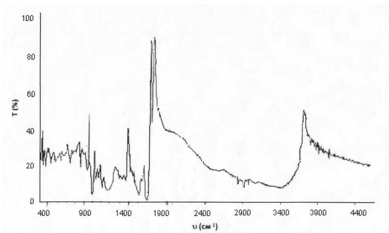
Рис.1. ИК-спектры гуминовых кислот, выделенных из угля Кызыл-Кия.
