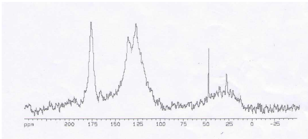
Рис.2. ^{13}\text{C} ЯМР спектры ГК (уголь Кызыл-Кия).
