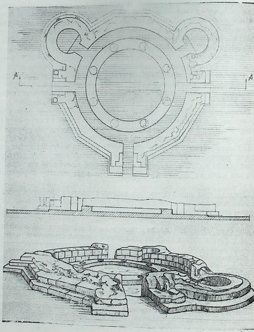
Рис. 1. Храм на горе Килисадаг (обмерный чертеж 1973 г.): а — общий вид; б — разрез А—А; в — план.
