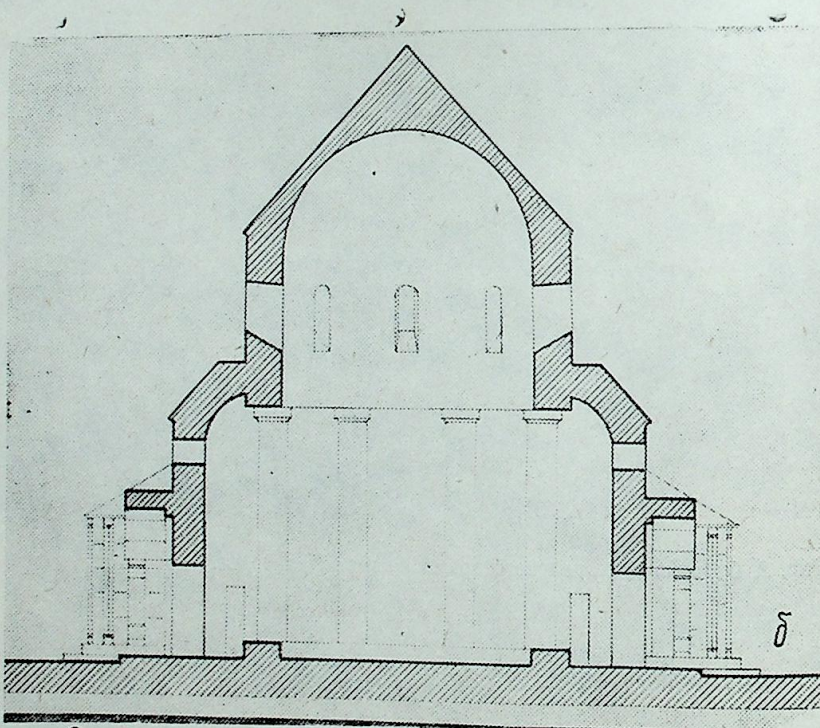
Рис. 3. К проекту реставрации храма на горе Килисадаг: а) главный фасад; б — разрез А—А.
