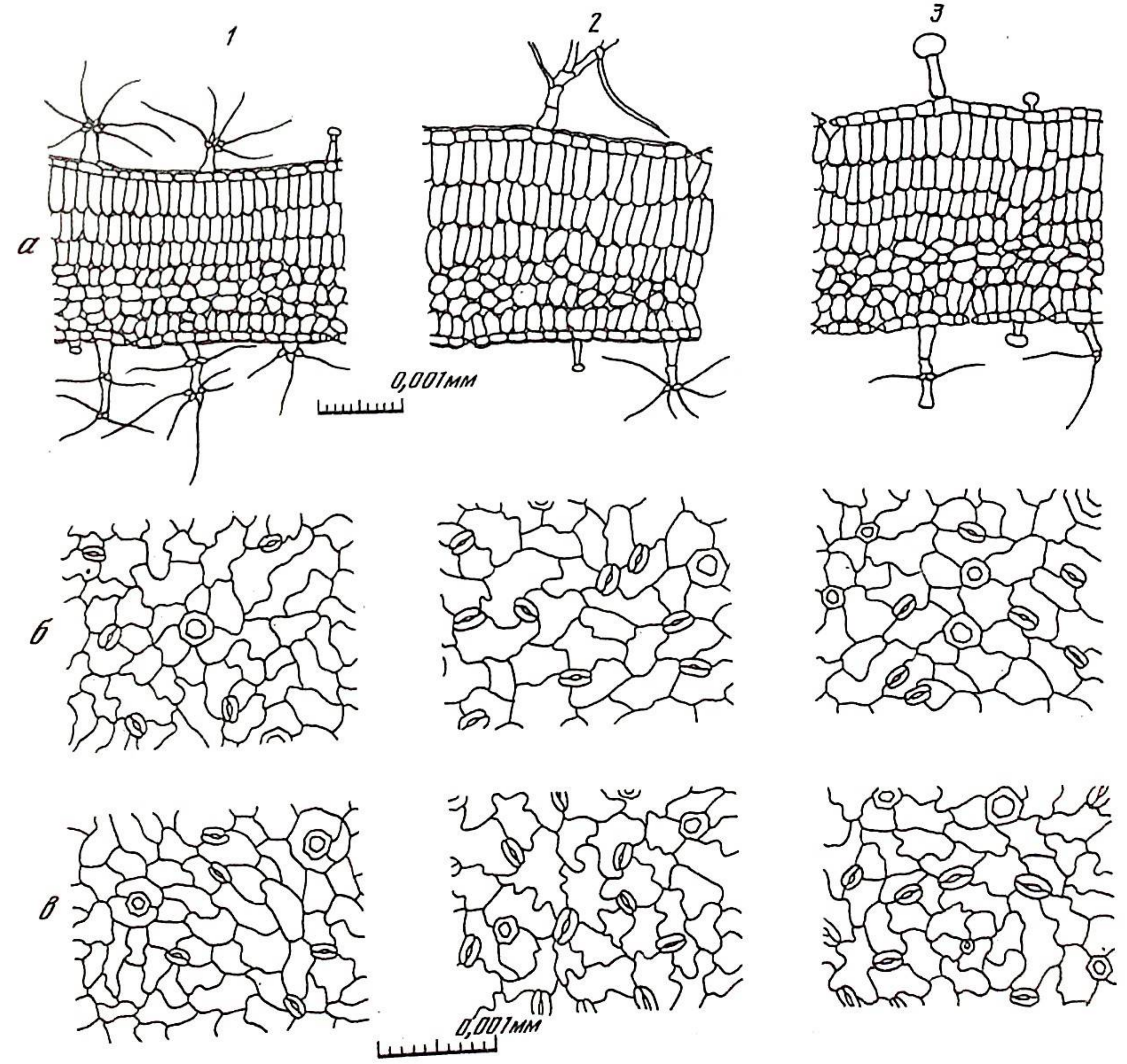
Рис. 4. Анатомическое строение листовой пластинки а — поперечный разрез, б — верхний эпидермис, в — нижний эпидермис; 1 — Verbascum phlomoides , 2 — V. pinnatifidum , 3 — V. phlomoides × V. pinnatifidum
