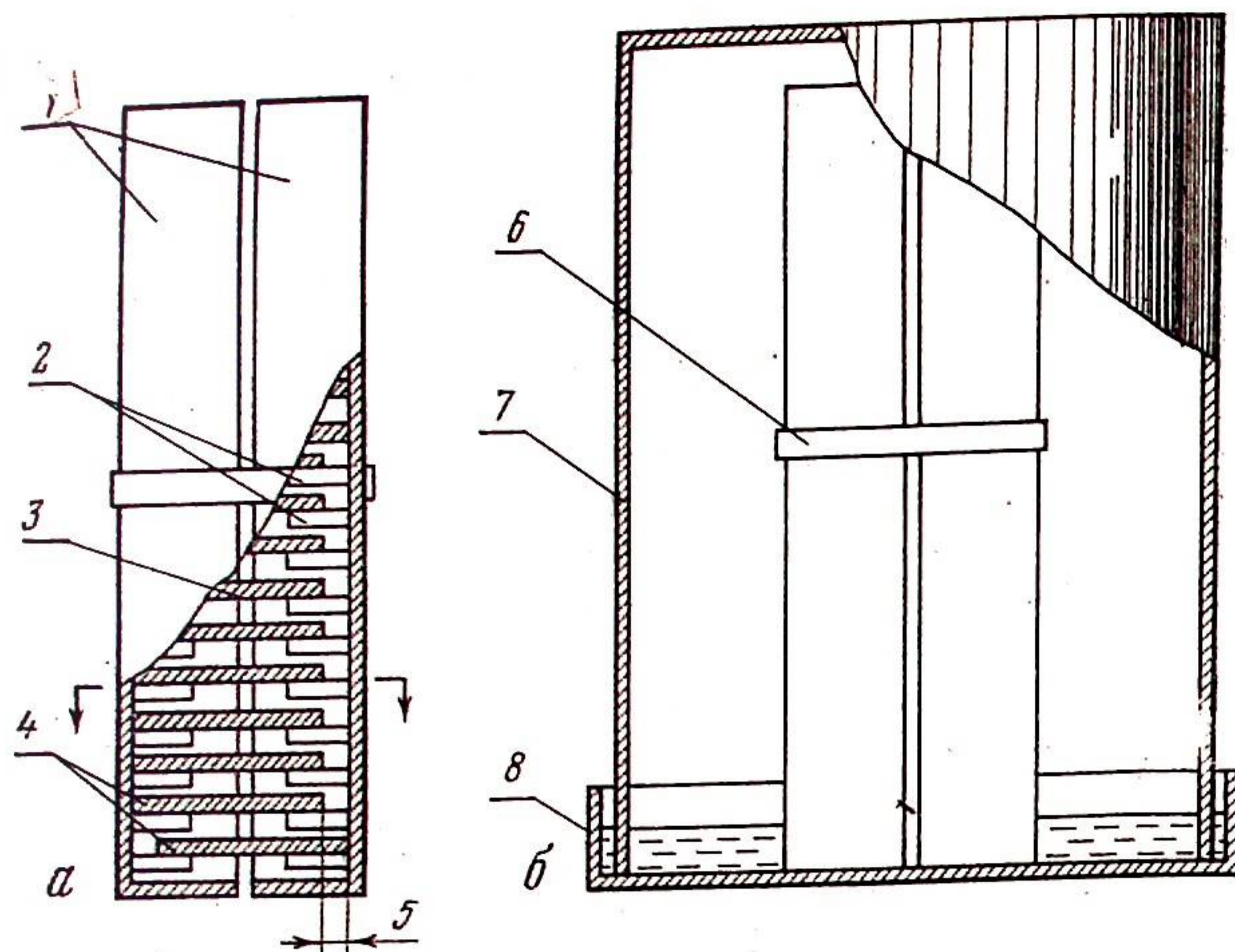
Рис. 2. Чертеж кассеты для проращивания пыльцы хвойных
