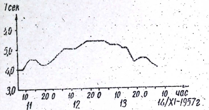
Рис. 6. Изменение периода микросейсм на вертикальной составляющей во время «бури микросейсм» 11—14 ноября 1957 г.
