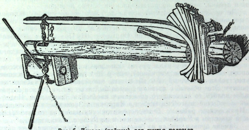
Рис. 5. Лекало (пайним) для гнуща полозьев
