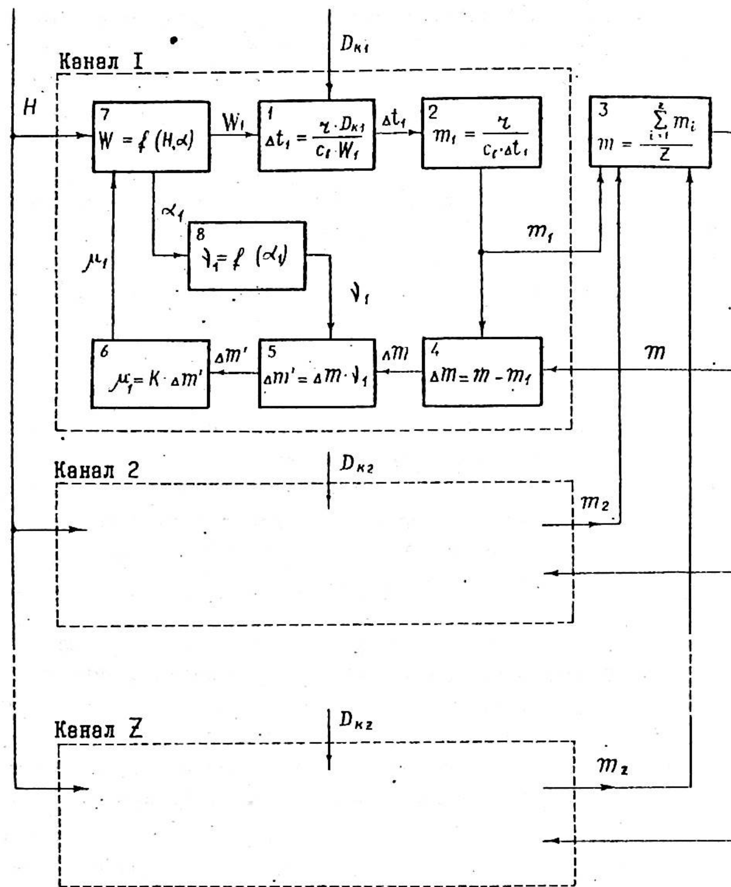
Рис. I. Функциональная схема системы управления.
