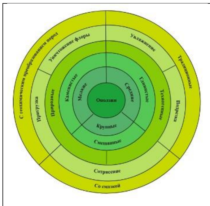
Рисунок 3. Типизация оползней
