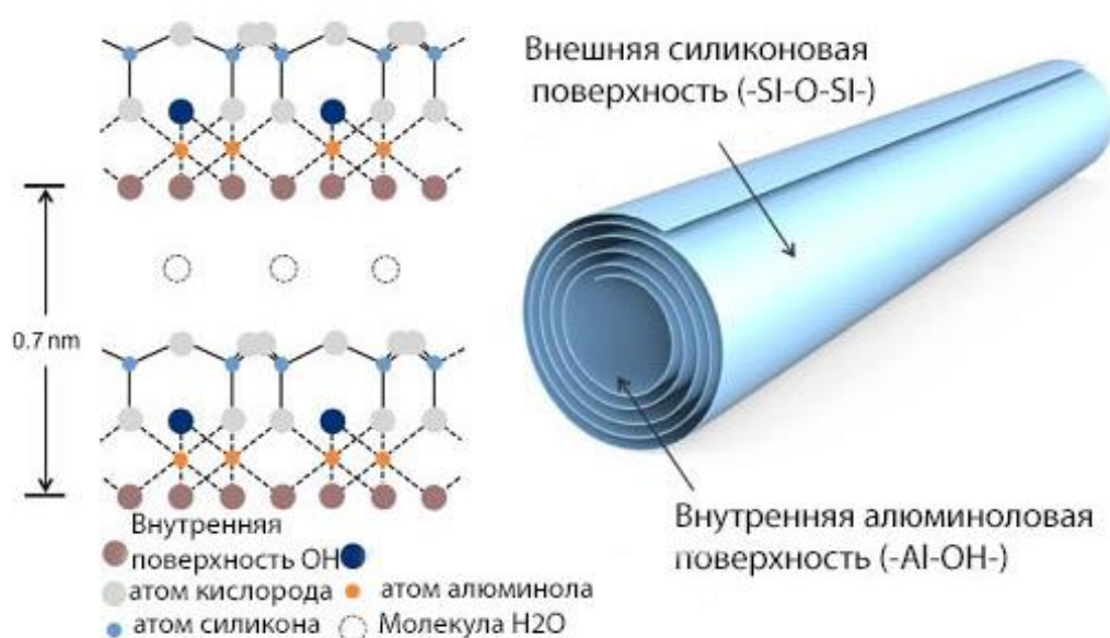
Рисунок 5. Схема строения галлуазитовой нанотрубки
